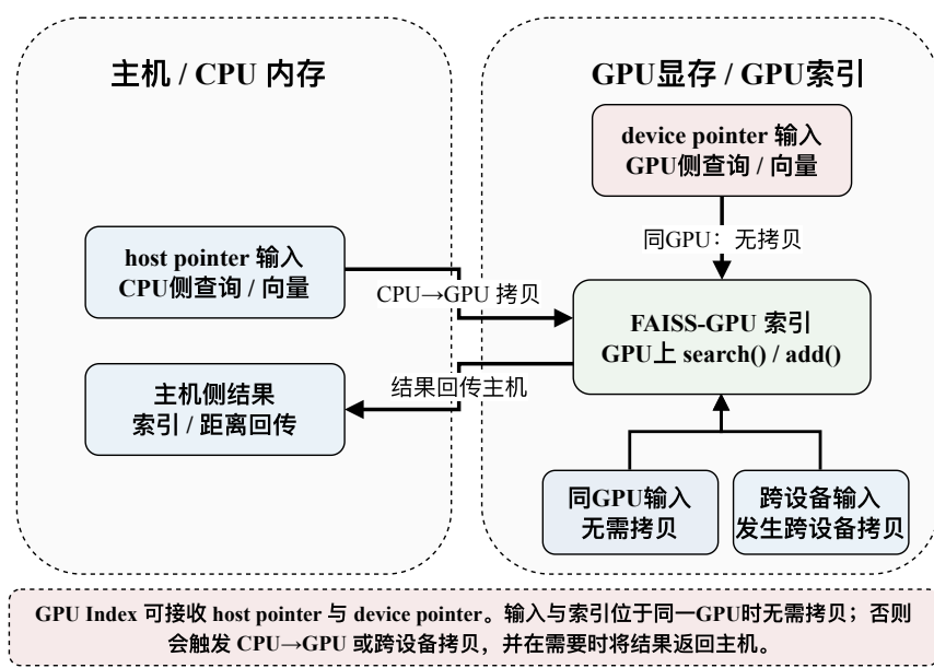
图 2-5 FAISS-GPU 的 CPU/GPU 互操作路径
