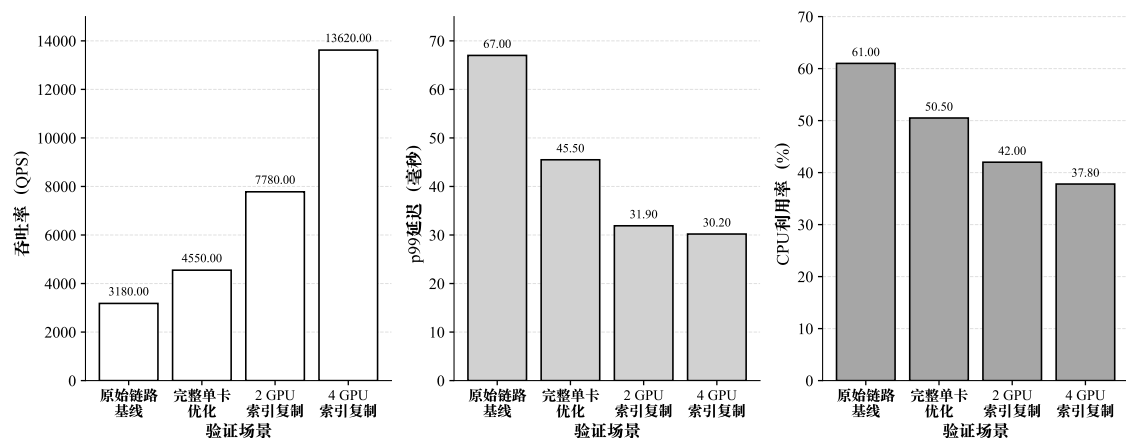
图 6-6 单卡优化与多 GPU 扩展收益对比
