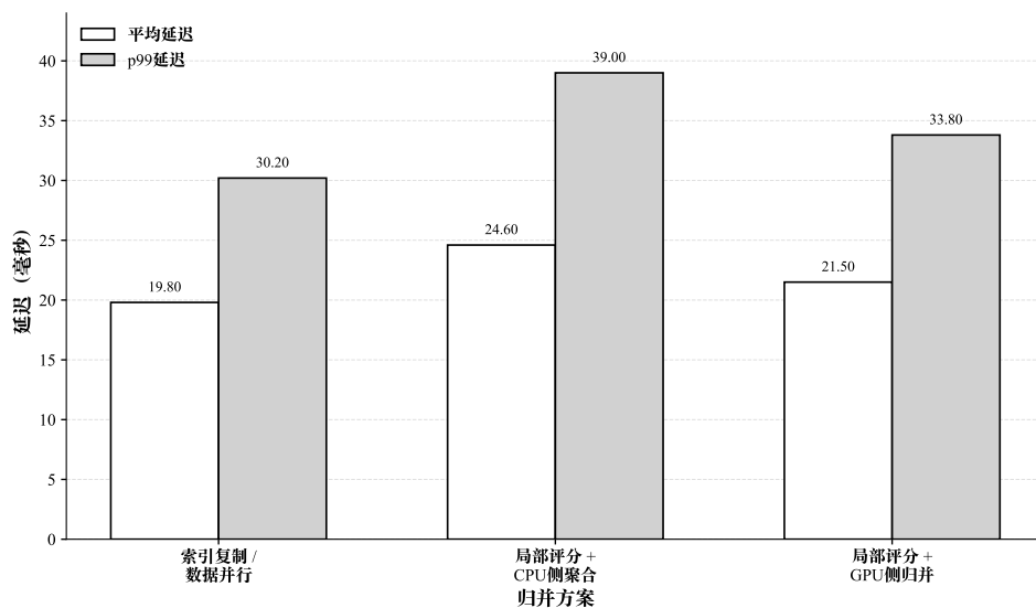
图 5-5 平均延迟与 p99 延迟变化
