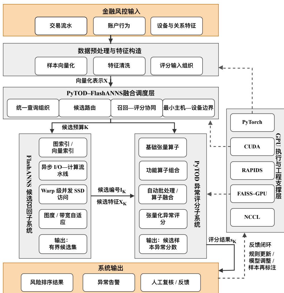
图 3-2 FlashTOD 系统概念图
