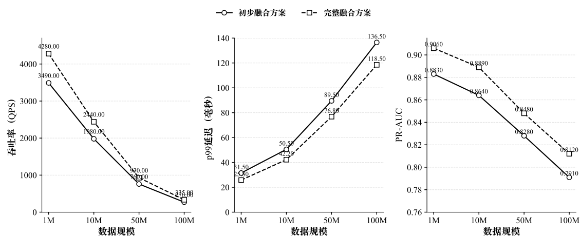
图 6-7 不同规模下系统表现趋势
