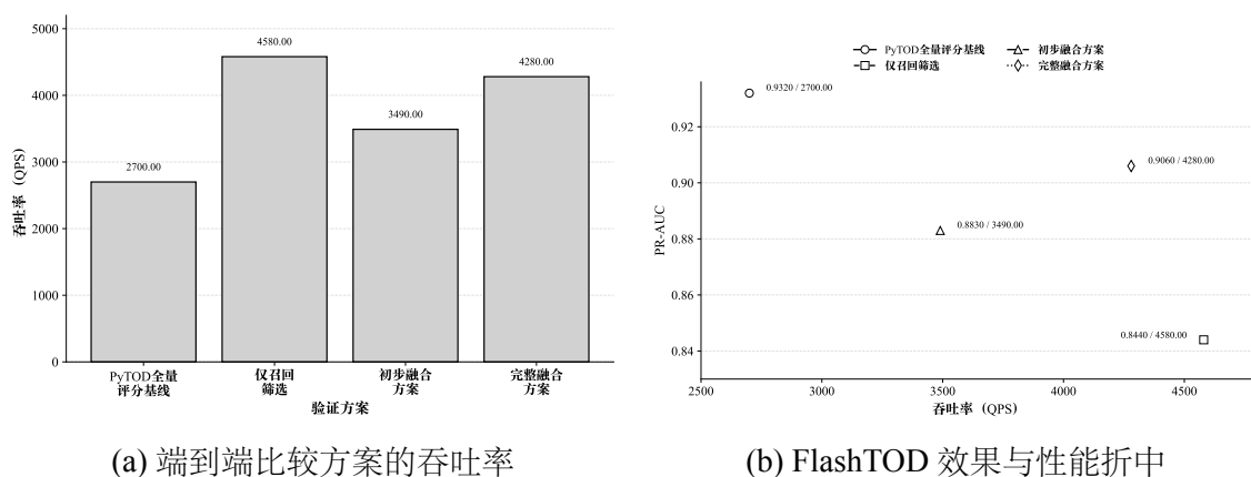
图 6-5 端到端比较方案的吞吐率与效果-性能折中
