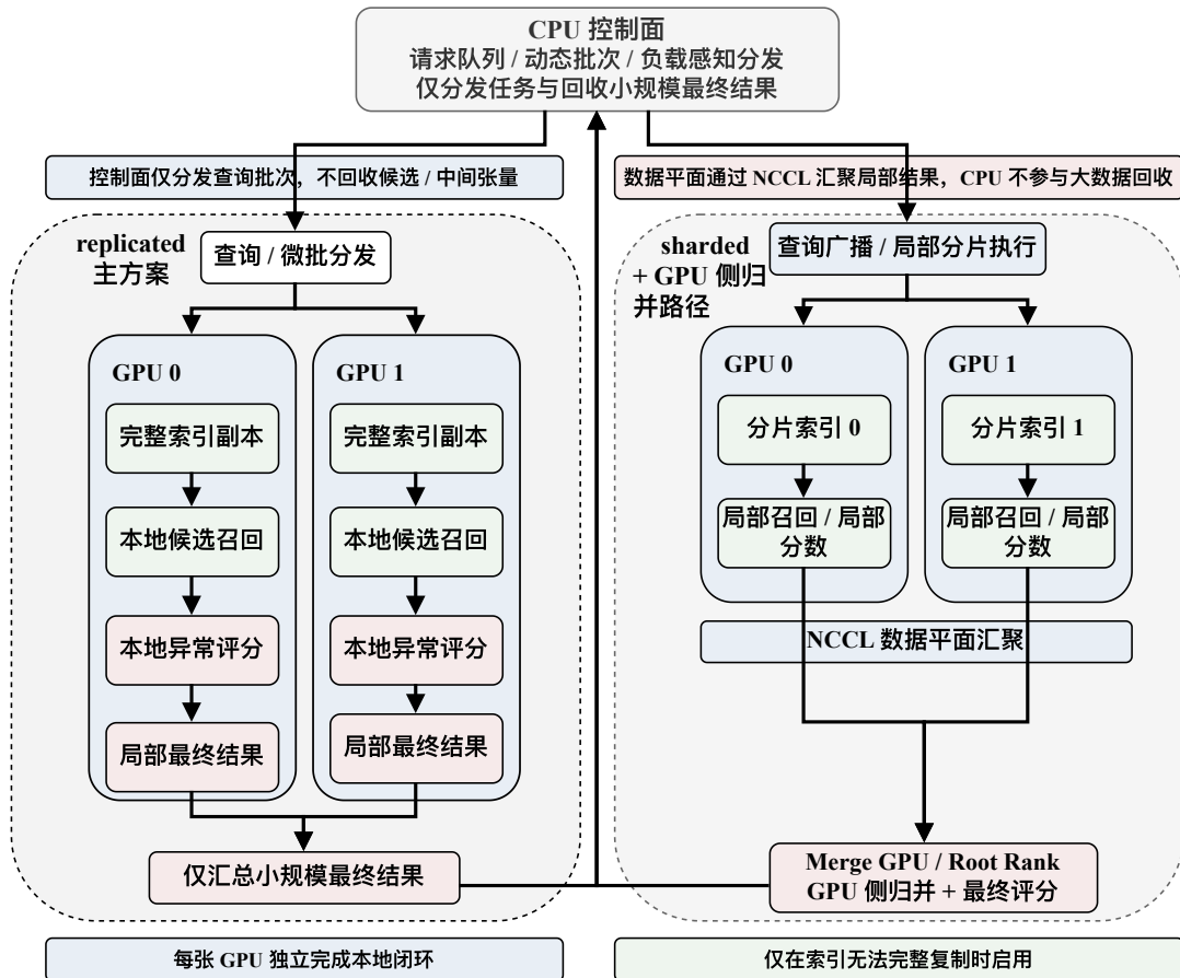
图 5-1 数据并行与索引复制多 GPU 架构
