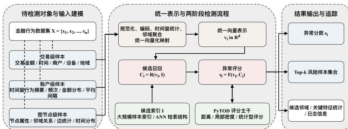
图 3-1 金融异常检测任务建模图
