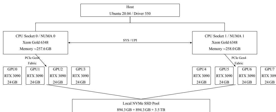
图 6-1 实验平台拓扑示意图
