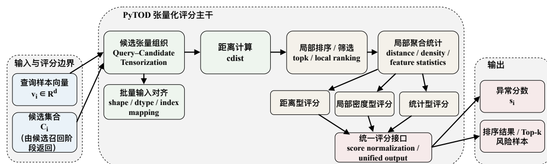
图 3-3 PyTOD 异常评分模块流程图
