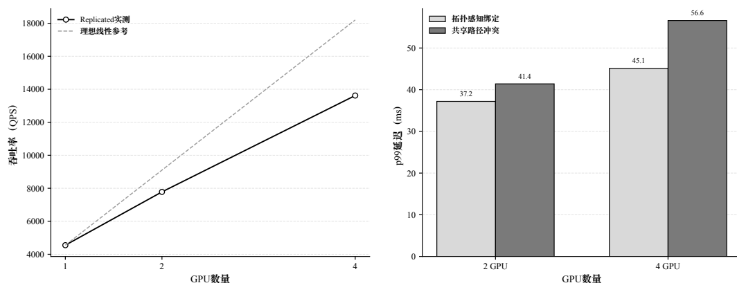
图 5-4 多 GPU 扩展趋势与共享路径瓶颈分析
