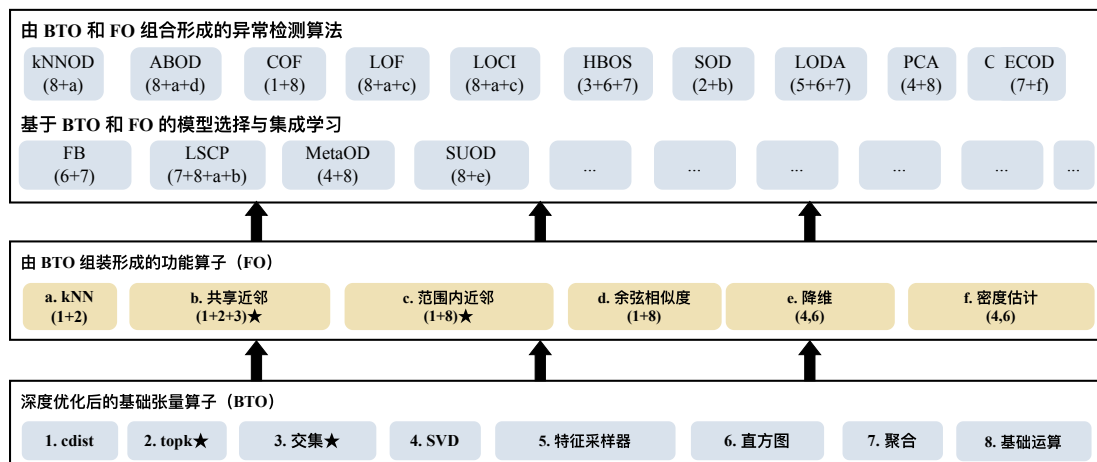
图 2-2 典型异常检测算法到张量算子的映射 [6]
