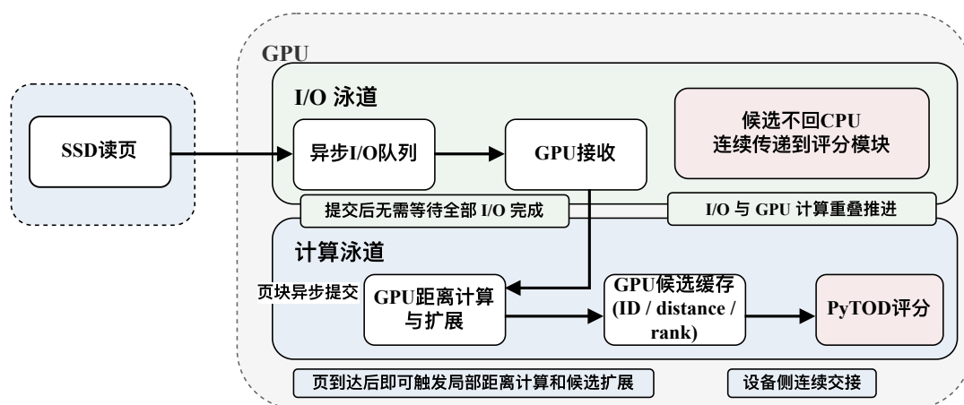
图 4-3 FlashANNS 异步 I/O—计算流水线与本文执行链路融合
