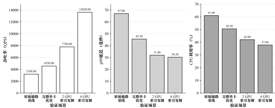
图 6-7 单卡优化与多 GPU 扩展收益对比
