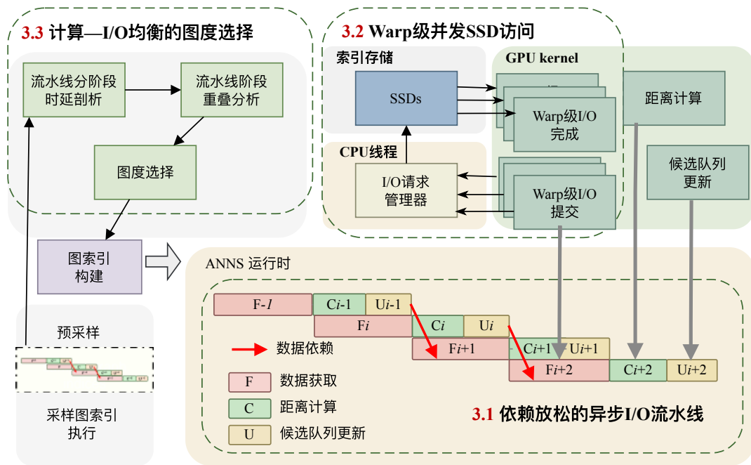
图 2-3 FlashANNS 异步 I/O—计算流水线原理 [7]
