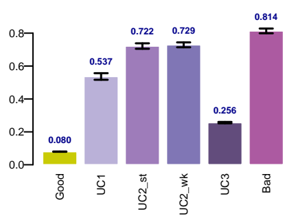
smape
