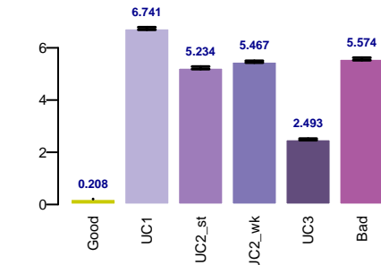
mape
