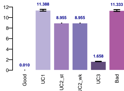
mae
