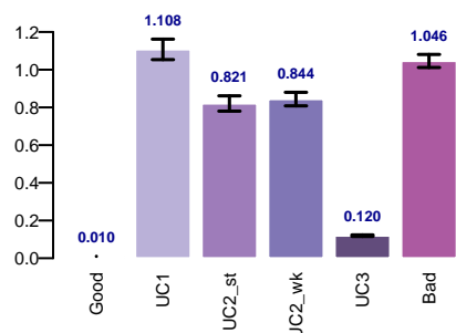
mae
