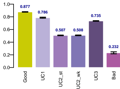
cn_smape
