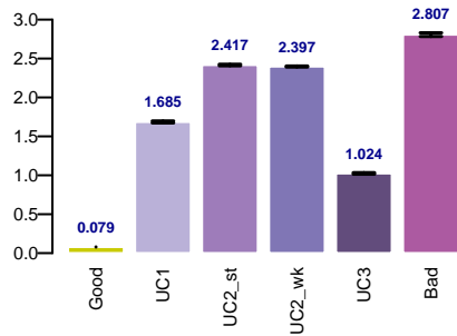
smape
