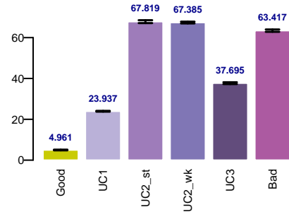
smape
