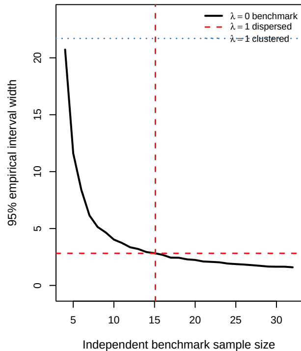
R2
