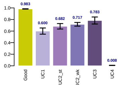
cn_smapc
