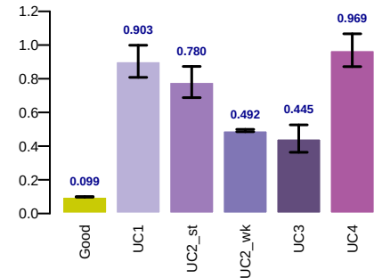
mape
