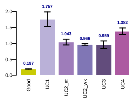
smape
