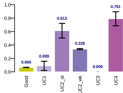
pic_mae
