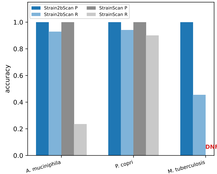
Precision / recall per species
