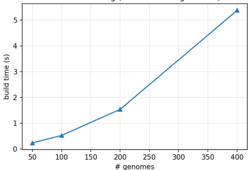
DB-build scaling (MinHash &gt;96 genomes)
