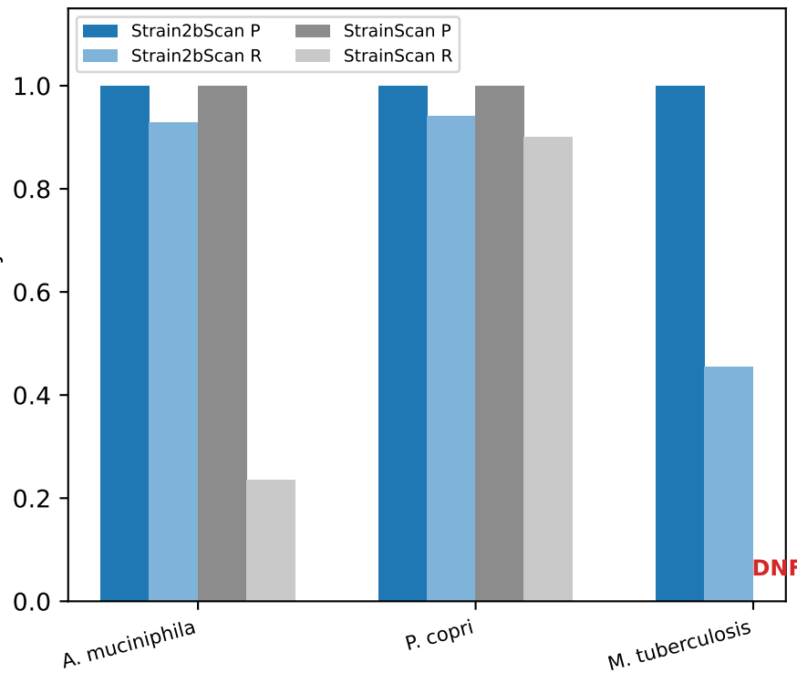
Precision / recall per species
