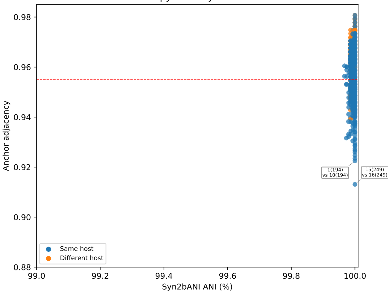
H. pylori — Syn2bANI
