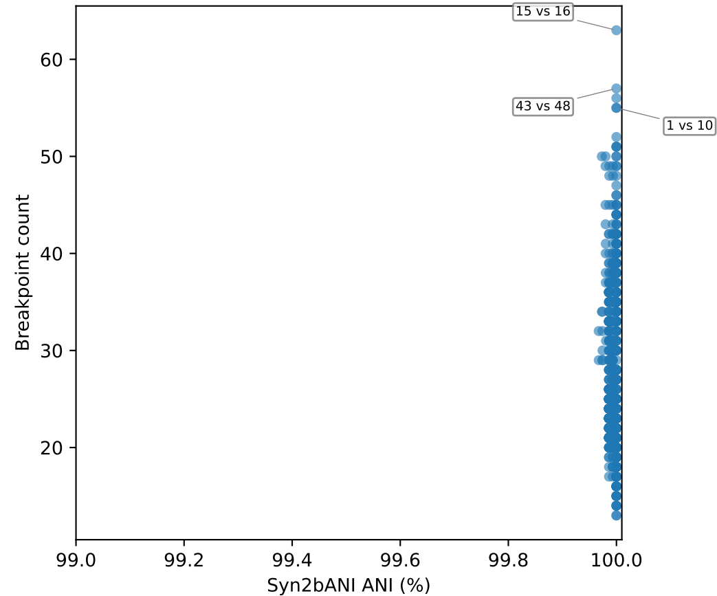
H. pylori
