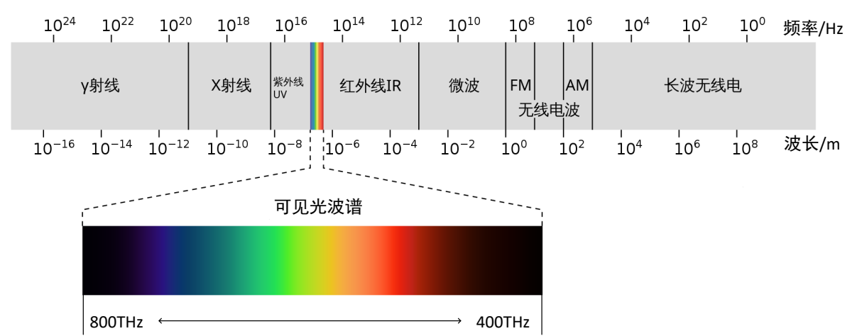
图 1-1 可见光波谱
