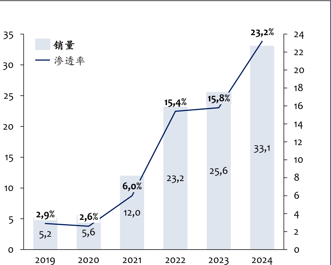
新能源物流车销量（万辆）及物流车新能源销量渗透率（%）
