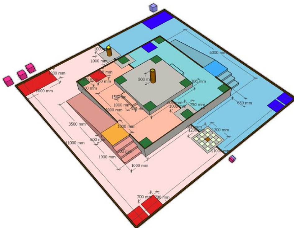
图 2 比赛场地尺寸（待改为俯视图）
