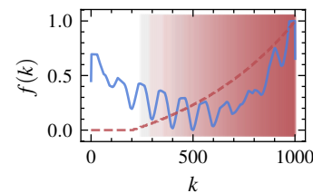
(s) PCA
