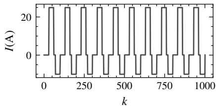
(d) LiSAD-GMM
