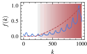
(h) EKF-NIS
