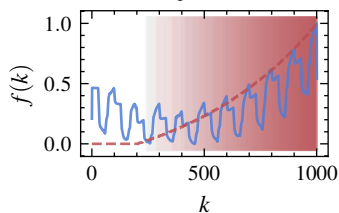
(n) OCSVM
