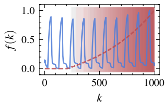
(j) AE
