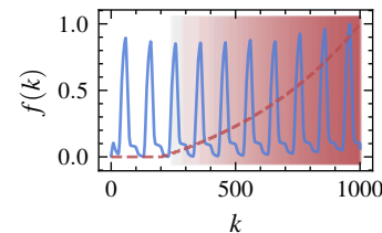
(k) LOF
