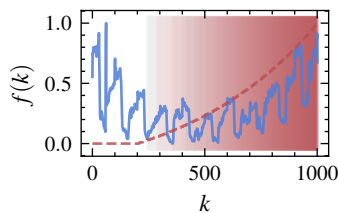
(q) USAD
