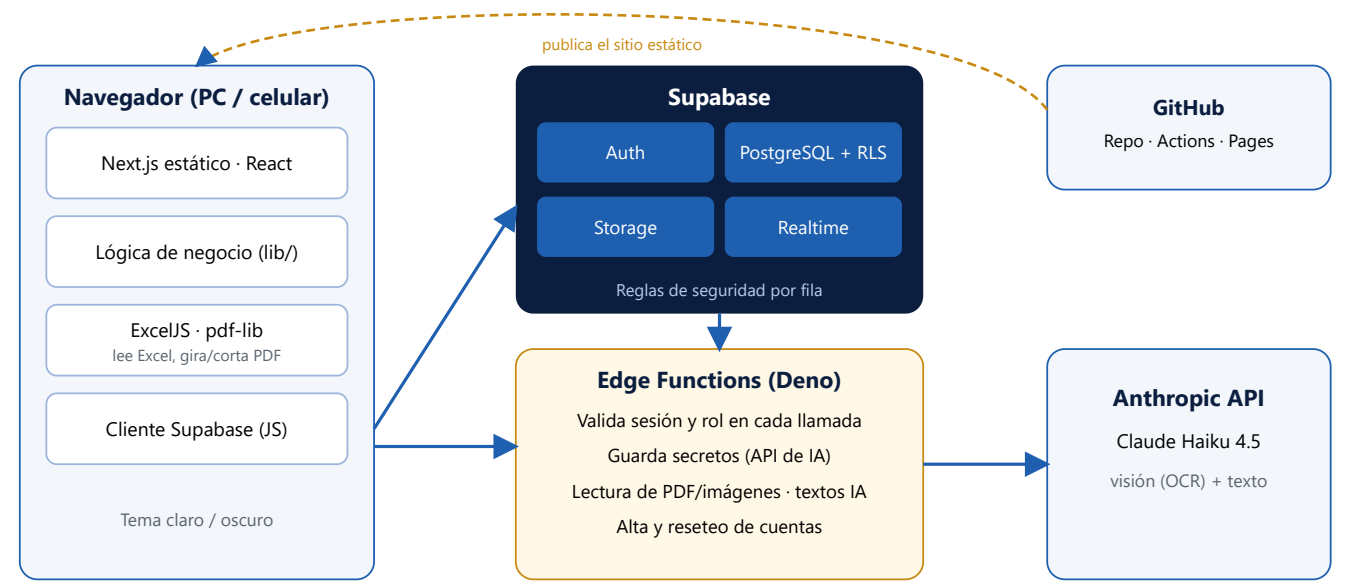
Figura 1. Componentes y flujo de datos.
