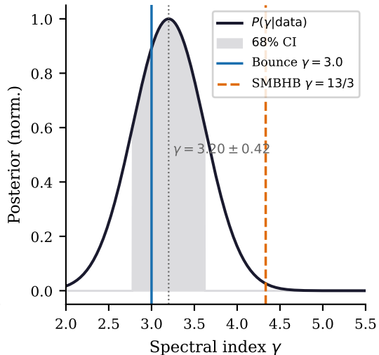
MCMC posterior
