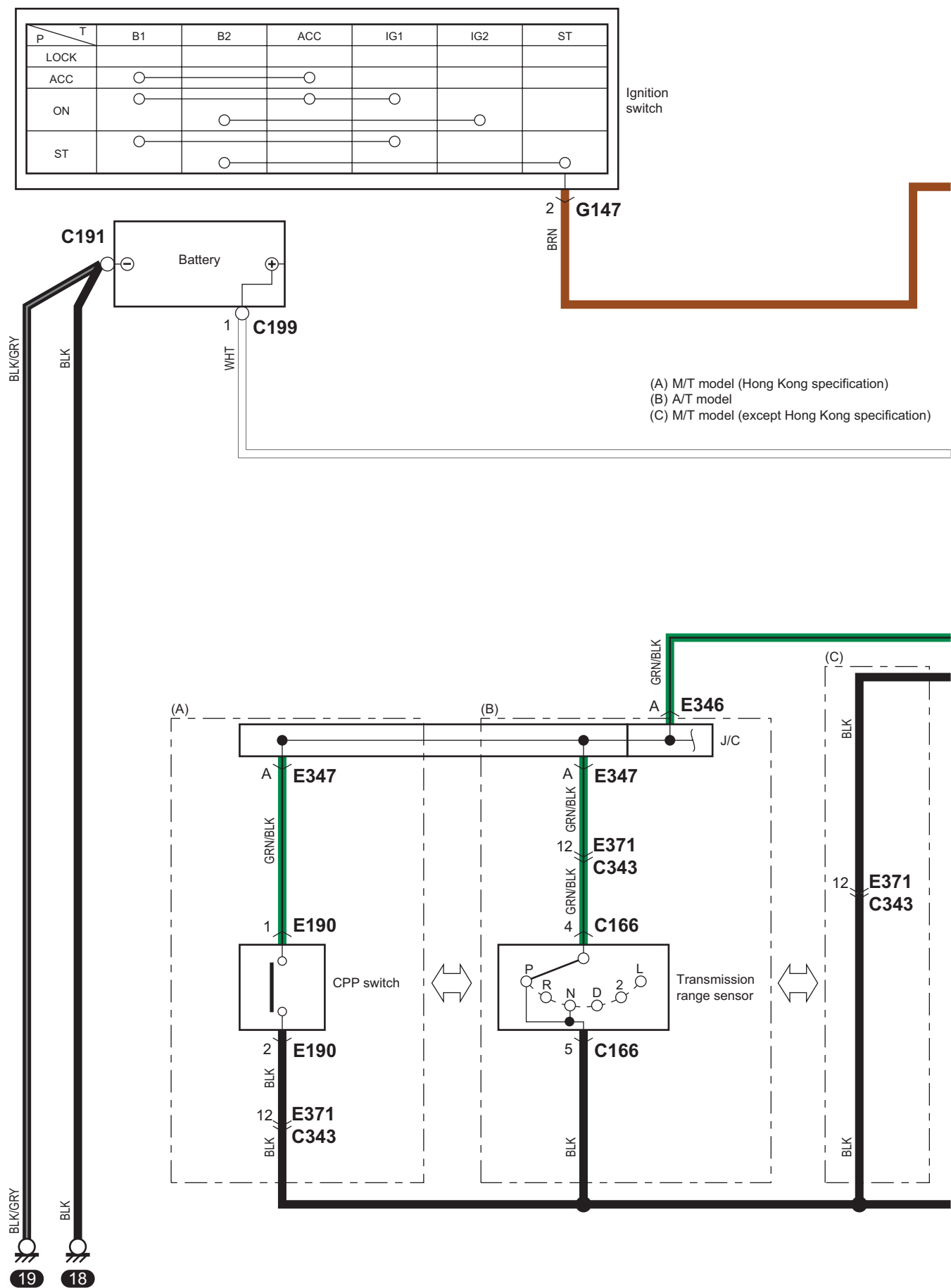
A-1-1 Diagrama del circuito del sistema de arranque (modelos de gasolina sin sistema de arranque por pulsación del motor)
