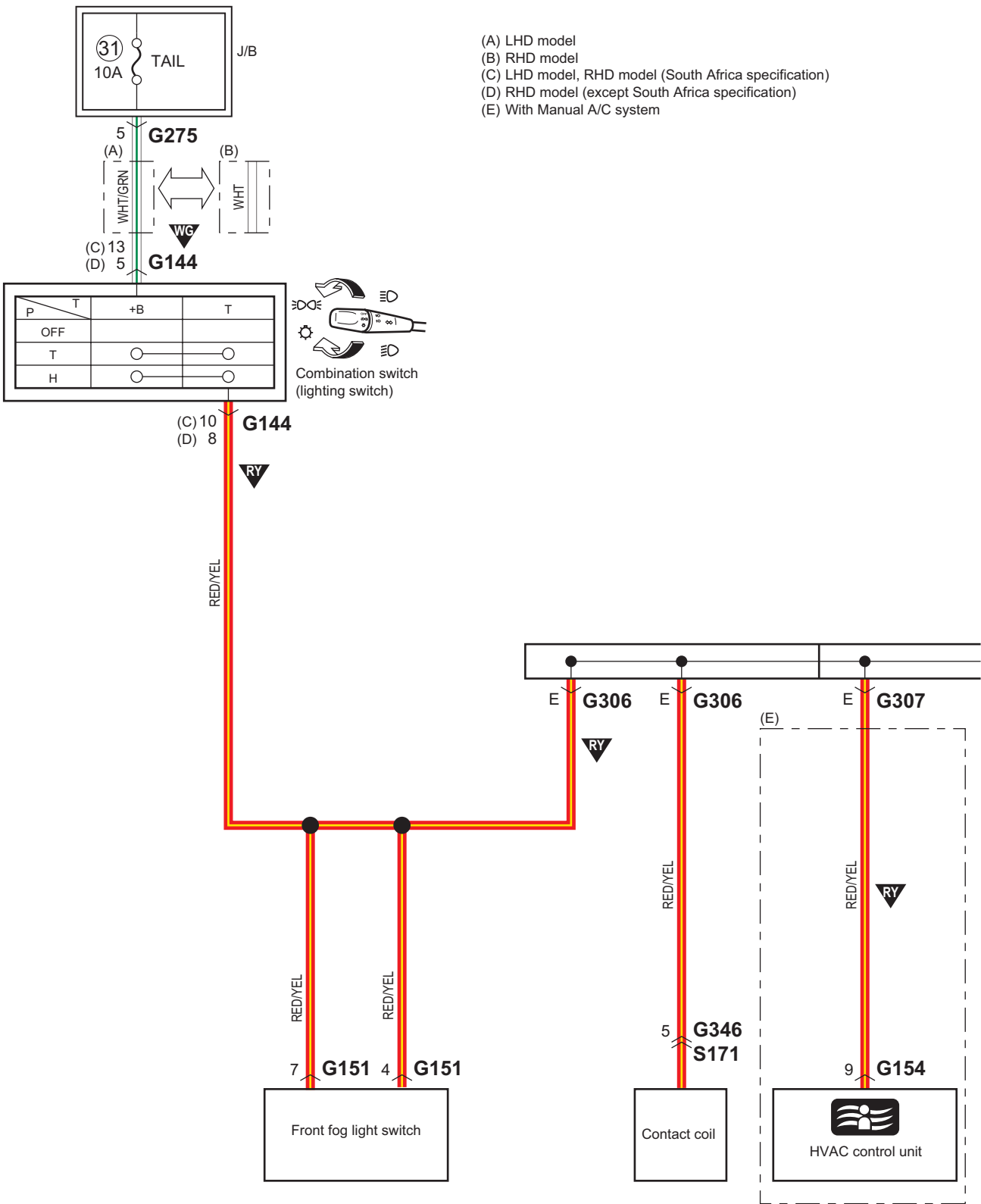
D-2-1 Diagrama del circuito del sistema de luz de la matrícula, de iluminación, de luces de posición y de luces traseras (sin sistema de arranque por pulsación del motor)
