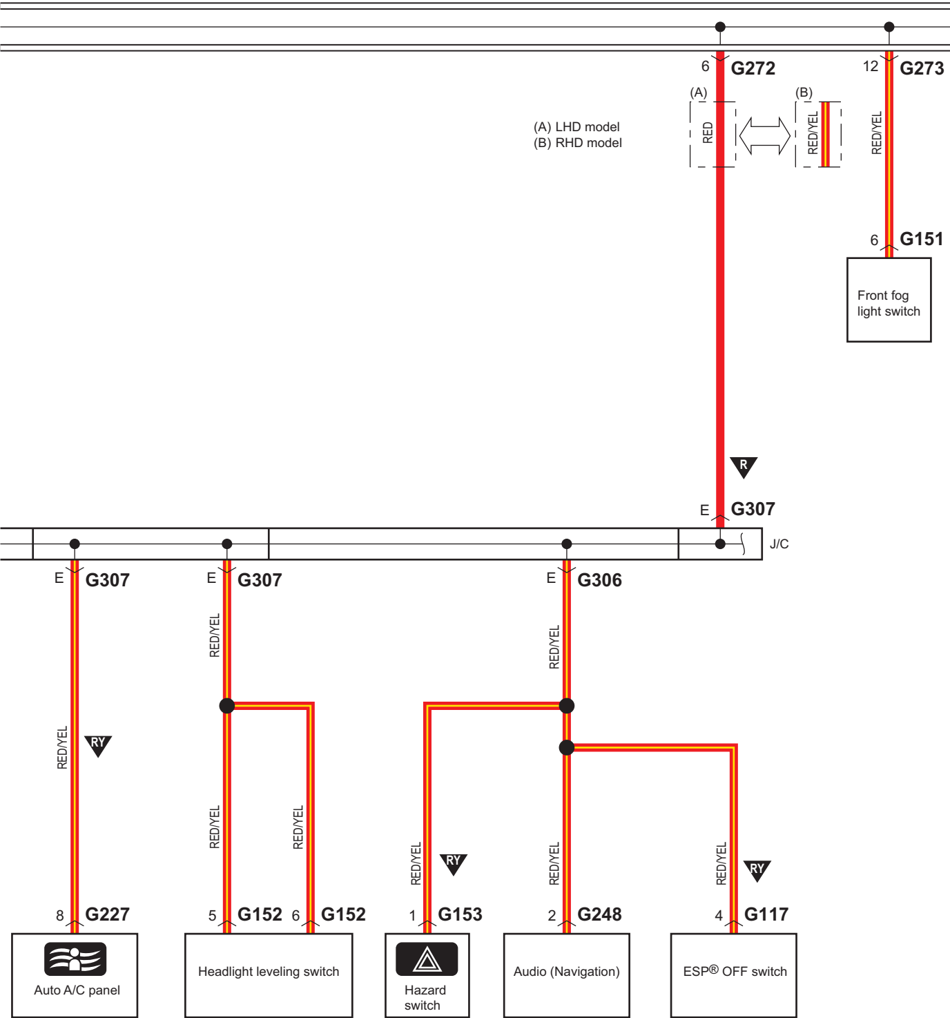
D-2-2 Diagrama del circuito del sistema de luz de la matrícula, de iluminación, de luces de posición y de luces traseras (con sistema de arranque por pulsación del motor)
