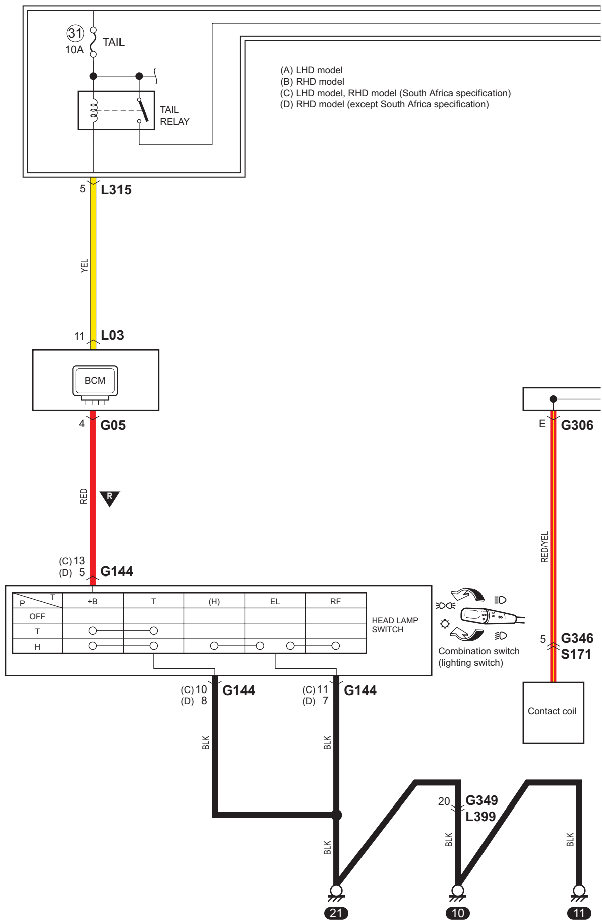
D-2-2 Diagrama del circuito del sistema de luz de la matrícula, de iluminación, de luces de posición y de luces traseras (con sistema de arranque por pulsación del motor)
