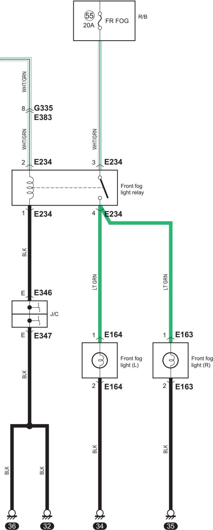
D-3-1 Diagrama del circuito del sistema de la luz antiniebla delantera (sin sistema de arranque por pulsación del motor)
