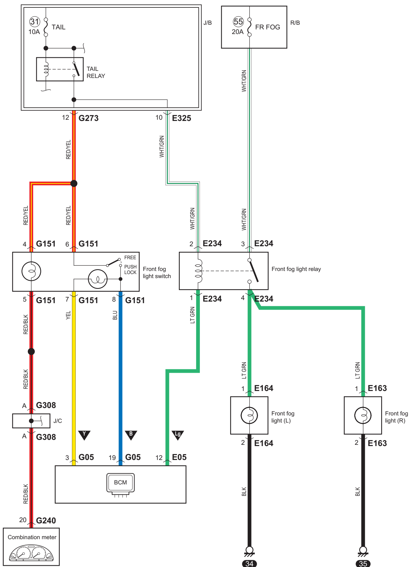
D-3-2 Diagrama del circuito del sistema de la luz antiniebla delantera (con sistema de arranque por pulsación del motor)
