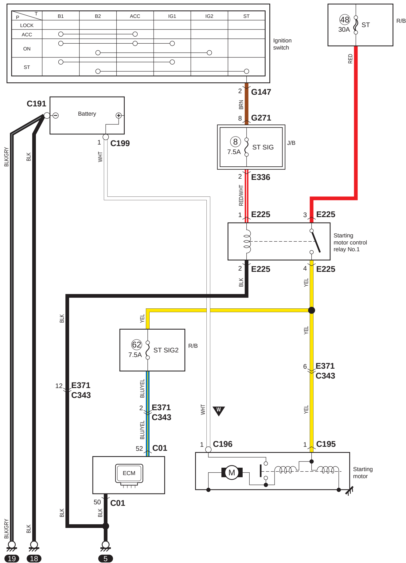
A-1-1 Shema kruga sustava za pokretanje (benzinski model bez sustava za pokretanje motora pritiskom prekidača)
