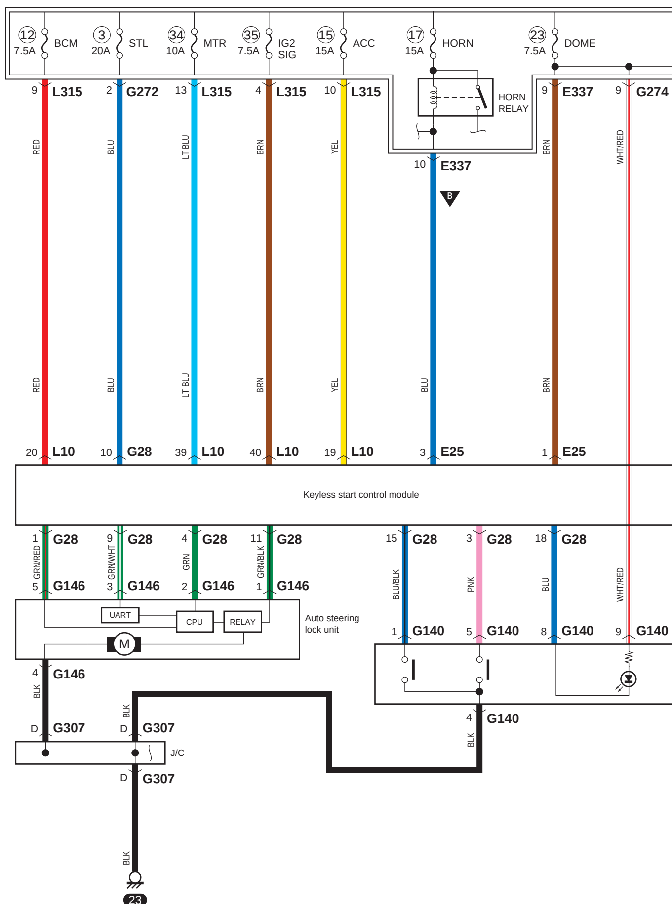
A-10 Shema kruga sustava upravljanja sigurnošću bez uporabe ključa (sa sustavom za pokretanje motora pritiskom prekidača)
