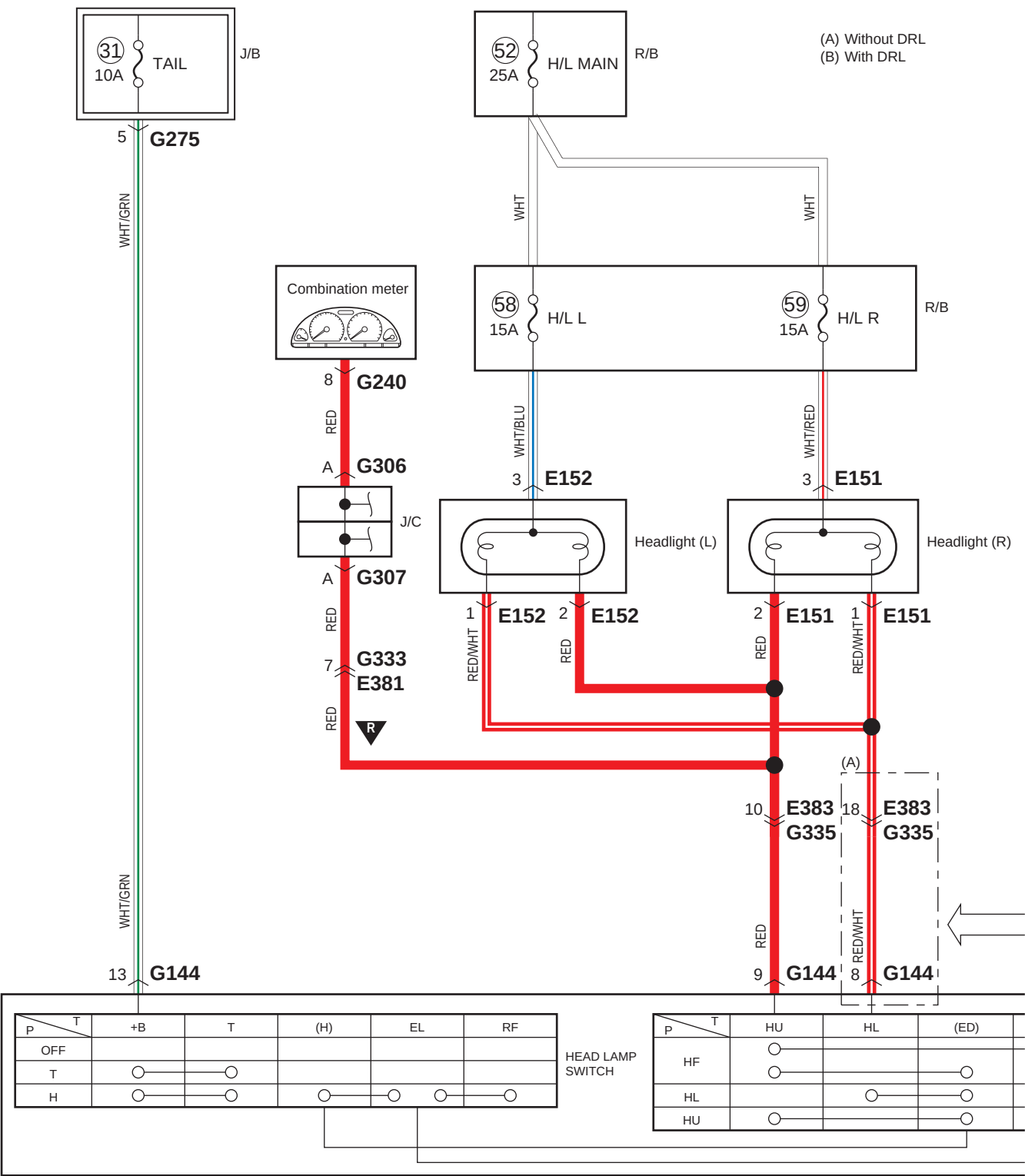
D-1-1 Shema kruga sustava prednjih svjetala (bez sustava za pokretanje motora pritiskom prekidača)
