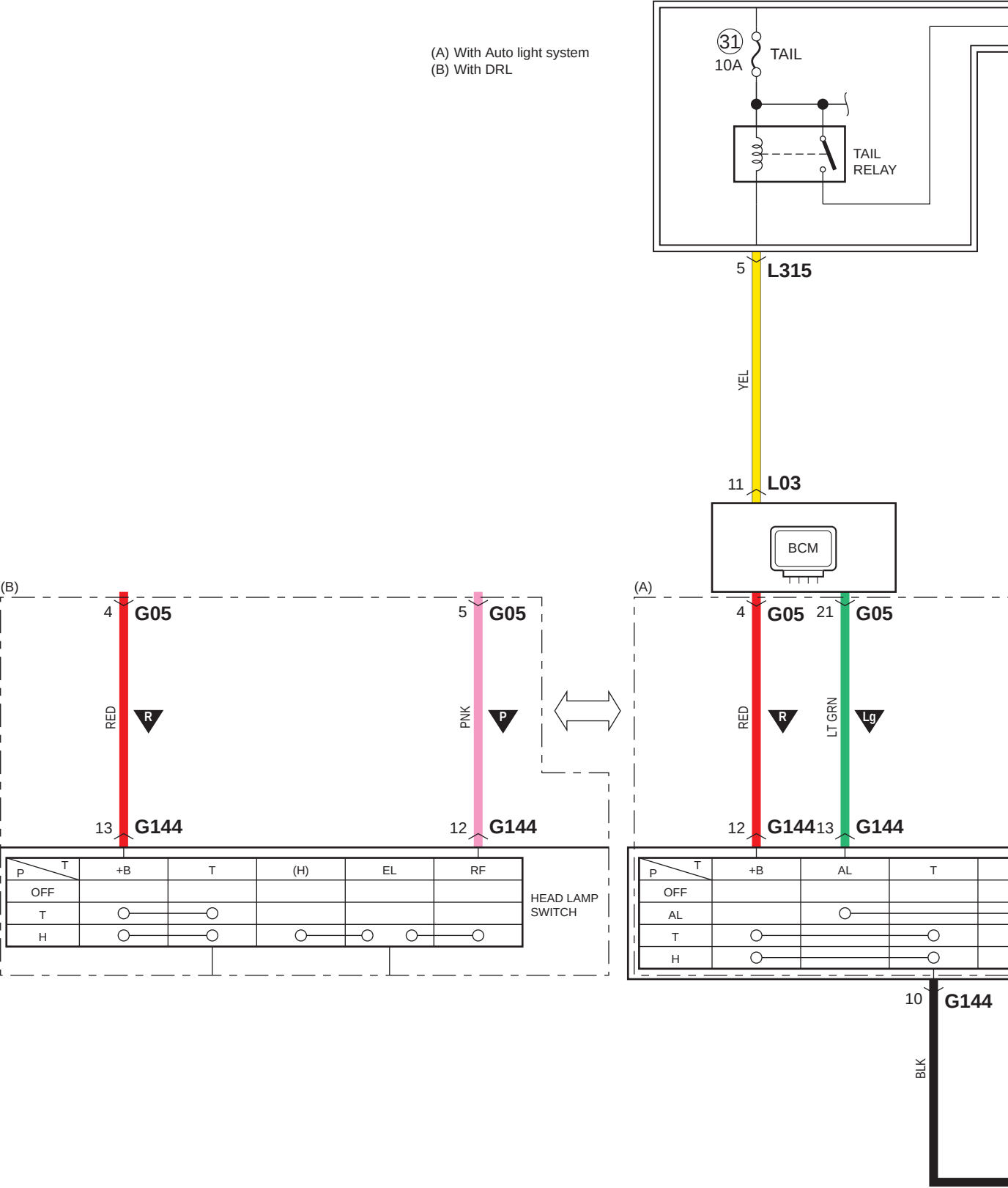
D-2-2 Shema kruga sustava pozicijskih i stražnjih svjetala, osvjetljenja i svjetla registarske pločice (sa sustavom za pokretanje motora pritiskom prekidača)
