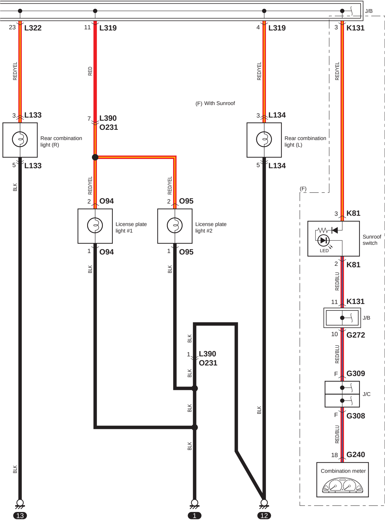
D-2-2 Shema kruga sustava pozicijskih i stražnjih svjetala, osvjetljenja i svjetla registarske pločice (sa sustavom za pokretanje motora pritiskom prekidača)
