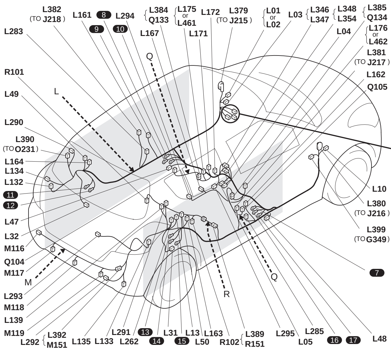
J/B BACK SIDE (LHD)
