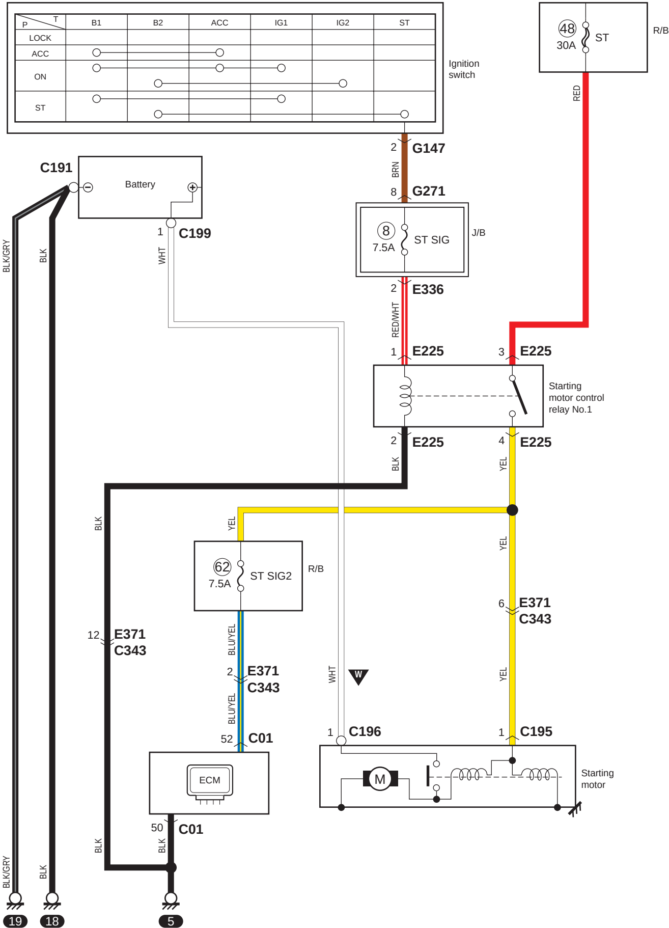
A-1-1 Schakelschema van het startsysteem (model met benzinemotor zonder motordrukknopstartstelsysteem)
