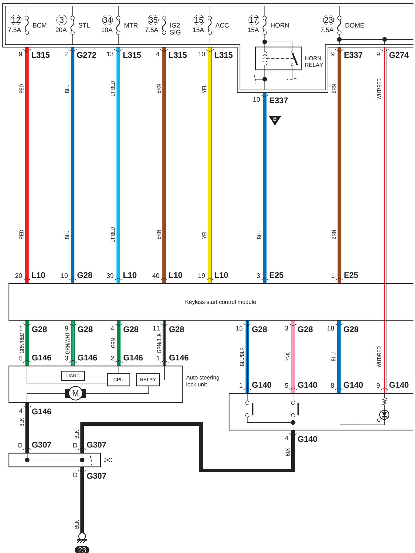
A-10 Schakelschema van het regelsysteem met beveiliging met afstandsbediening (met drukknopstartstelsel)
