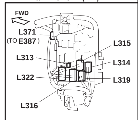
J/B BACK SIDE (LHD)
