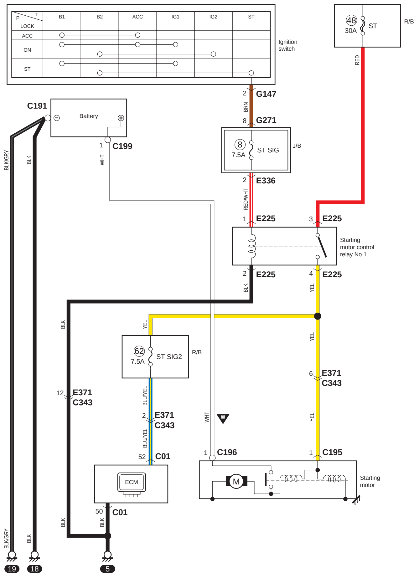
A-1-1 Schéma du circuit de système de lancement (modèle à essence sans système de démarrage du moteur)
