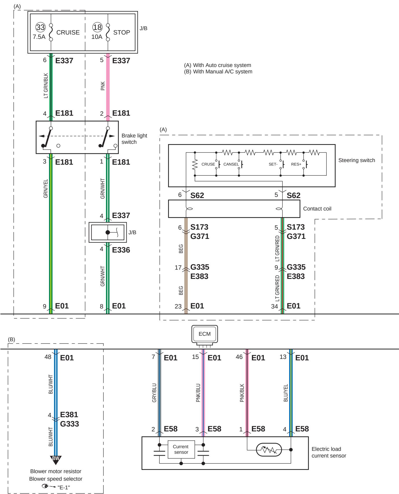
A-5-1 Schéma du circuit de système de commande A/C et moteur (modèle à essence)
