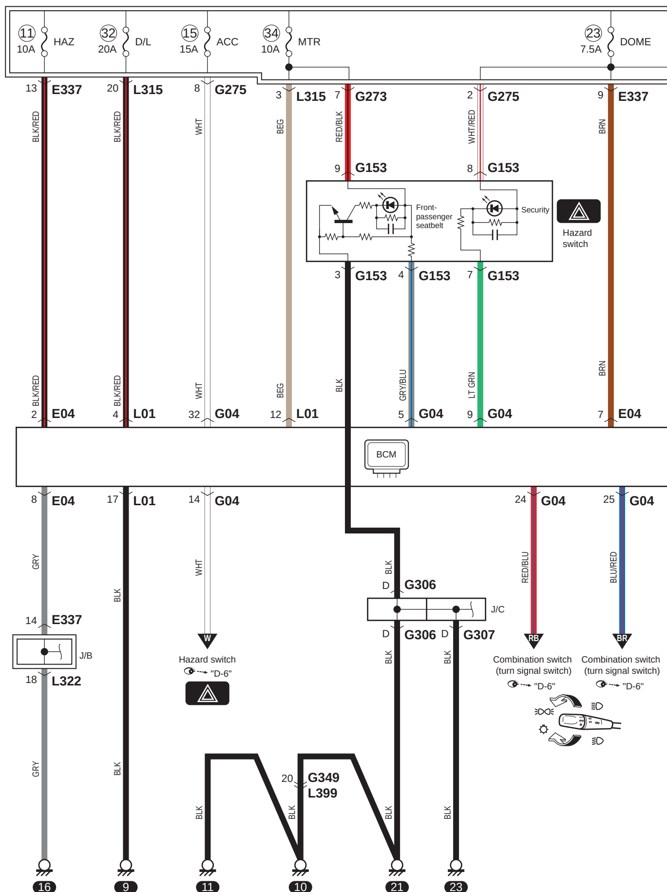
A-8-1 Schéma du circuit de système de commande de carrosserie (sans système de démarrage du moteur)
