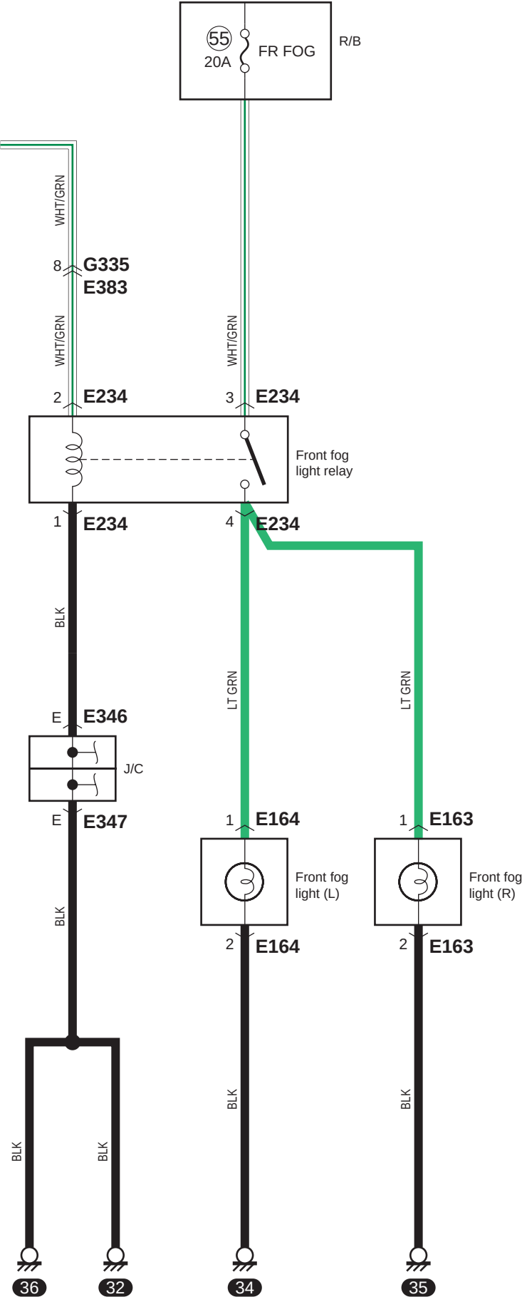
D-3-1 Schéma du circuit de système de feu antibrouillard avant (sans système de démarrage du moteur)
