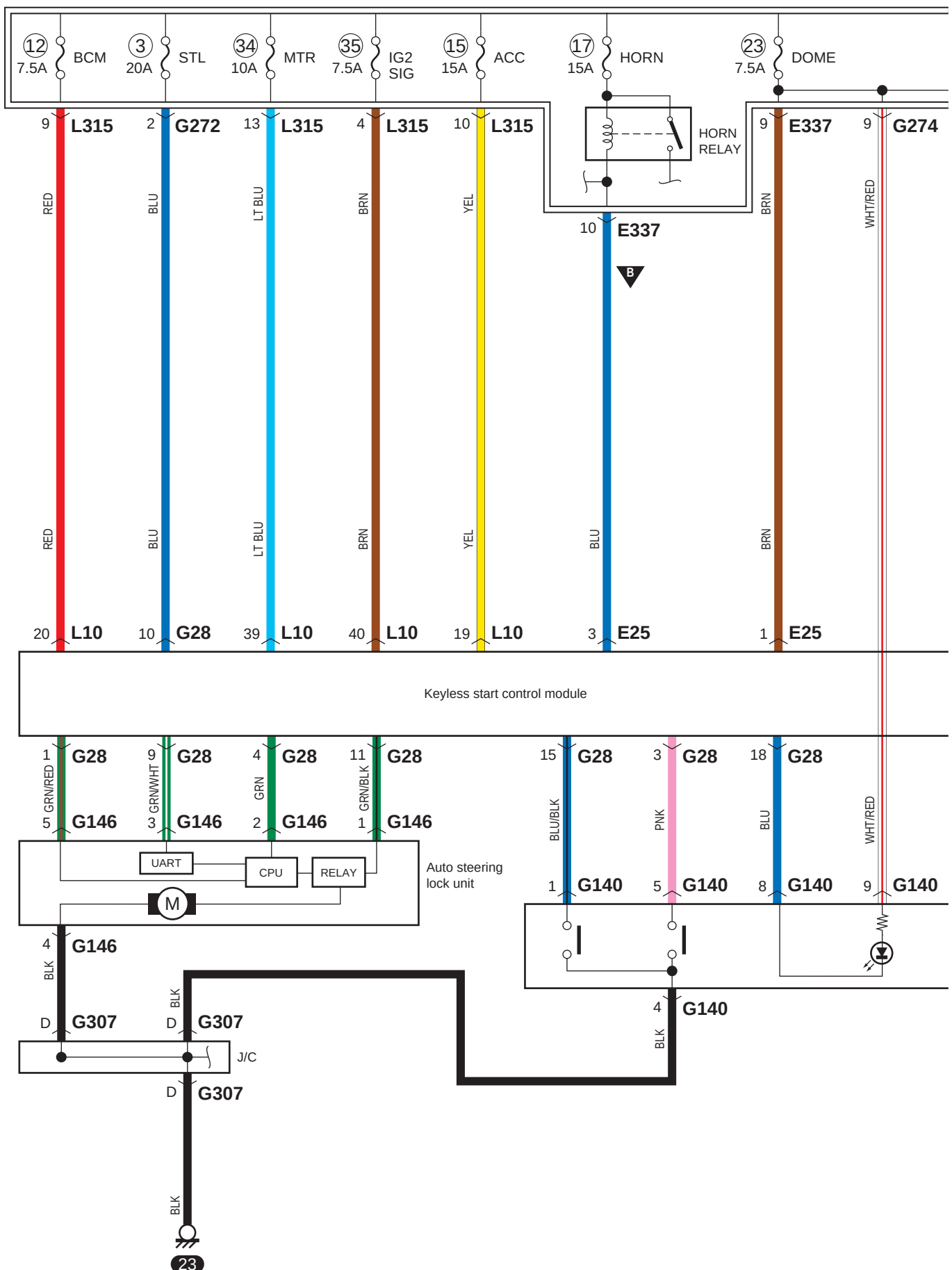
A-10 Διάγραμμα κυκλώματος συστήματος ελέγχου ασφάλειας χωρίς κλειδιά (Με σύστημα με μπουτόν εκκίνησης κινητήρα)
