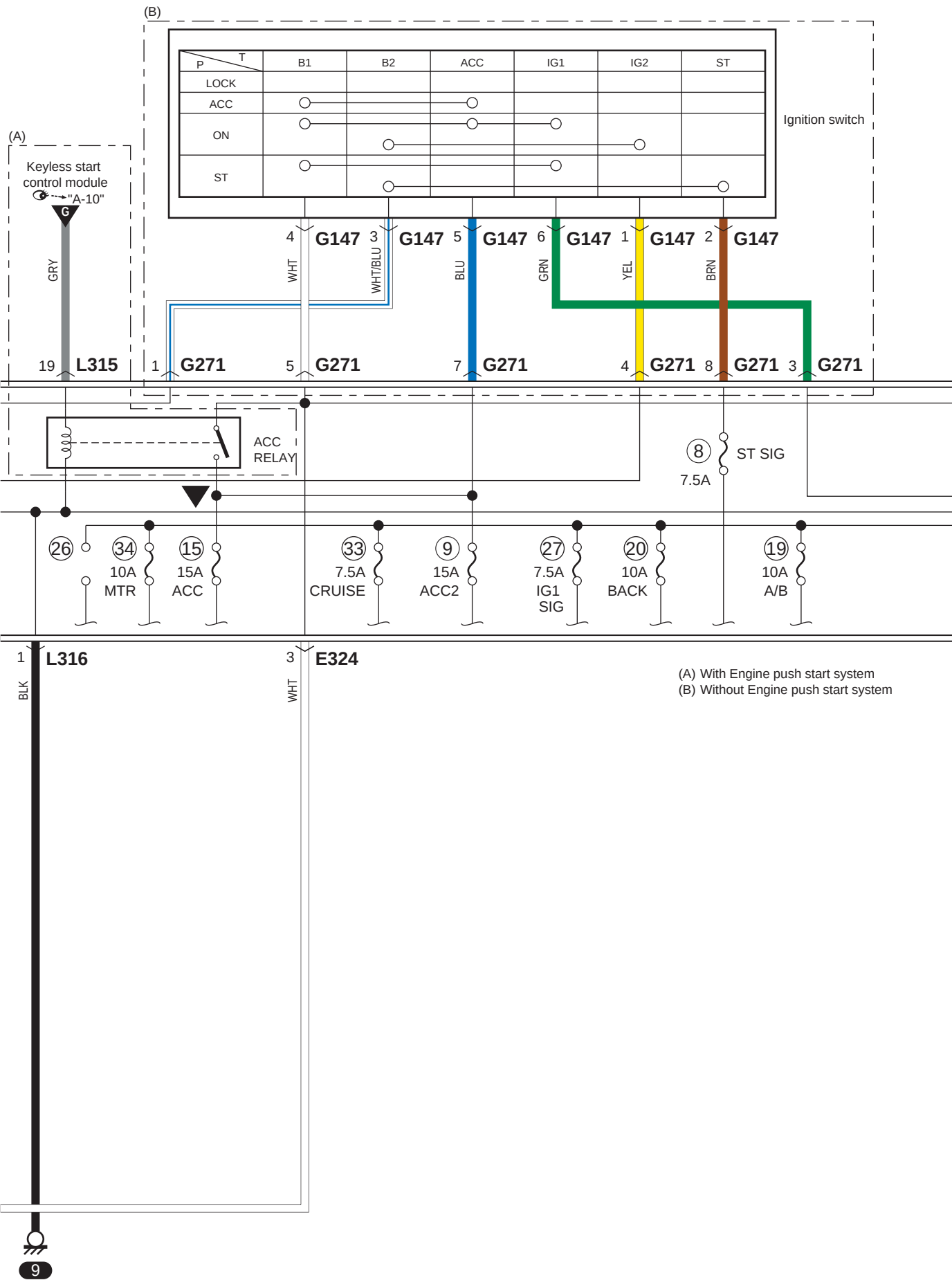
P-1-1 Tápellátás kapcsolási rajza (benzines modell)
