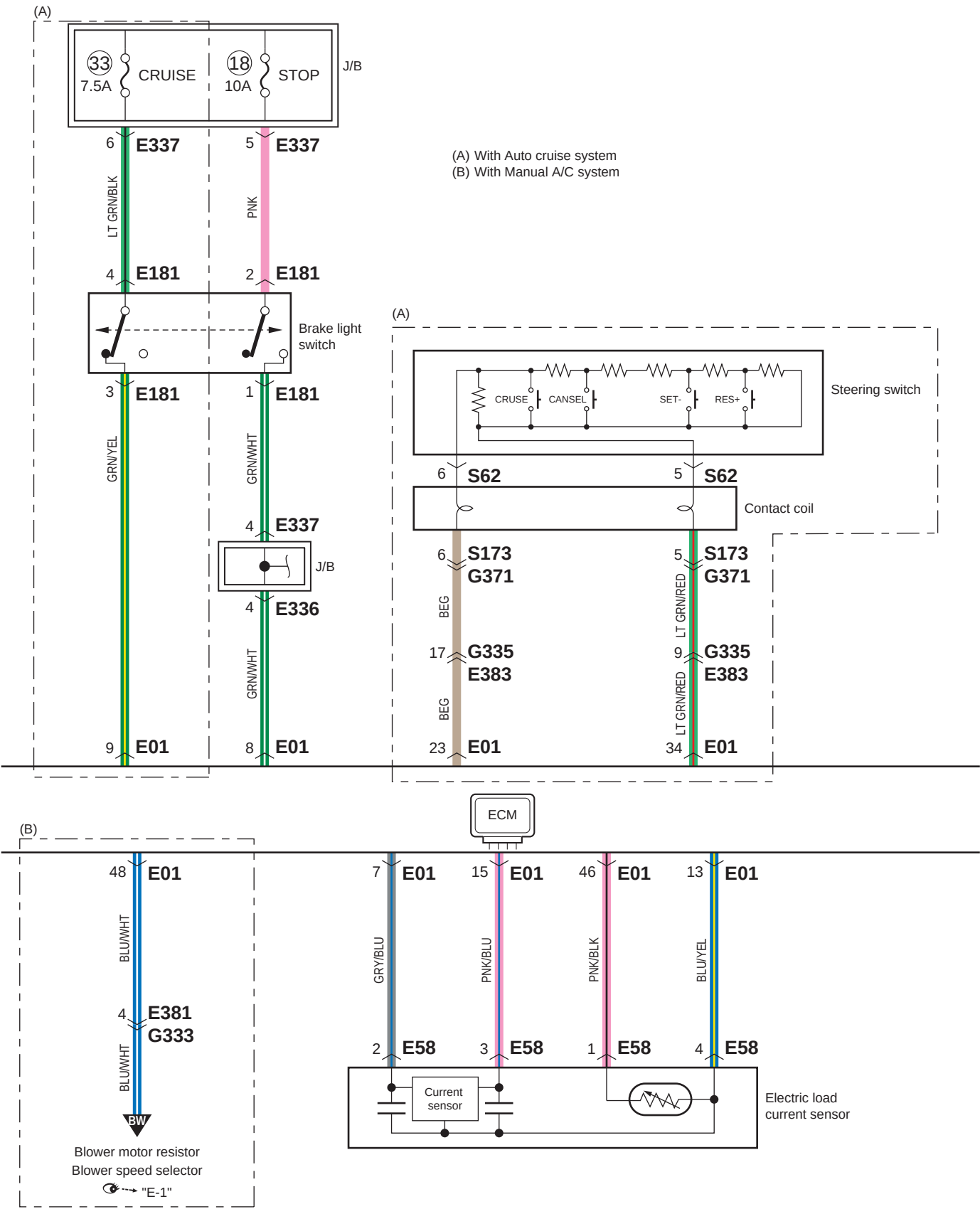
A-5-1 Motor és A/C vezérlőrendszer kapcsolási rajza (benzines modell)
