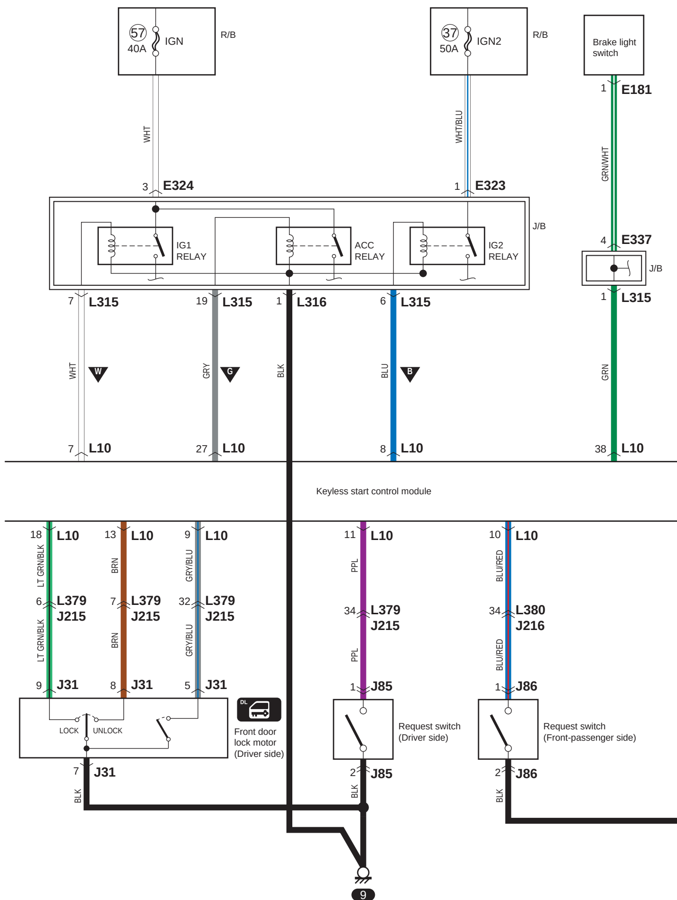
A-10 Kulcsnélküli biztonsági vezérlőrendszer kapcsolási rajza (nyomógombos motorindító rendszerrel)
