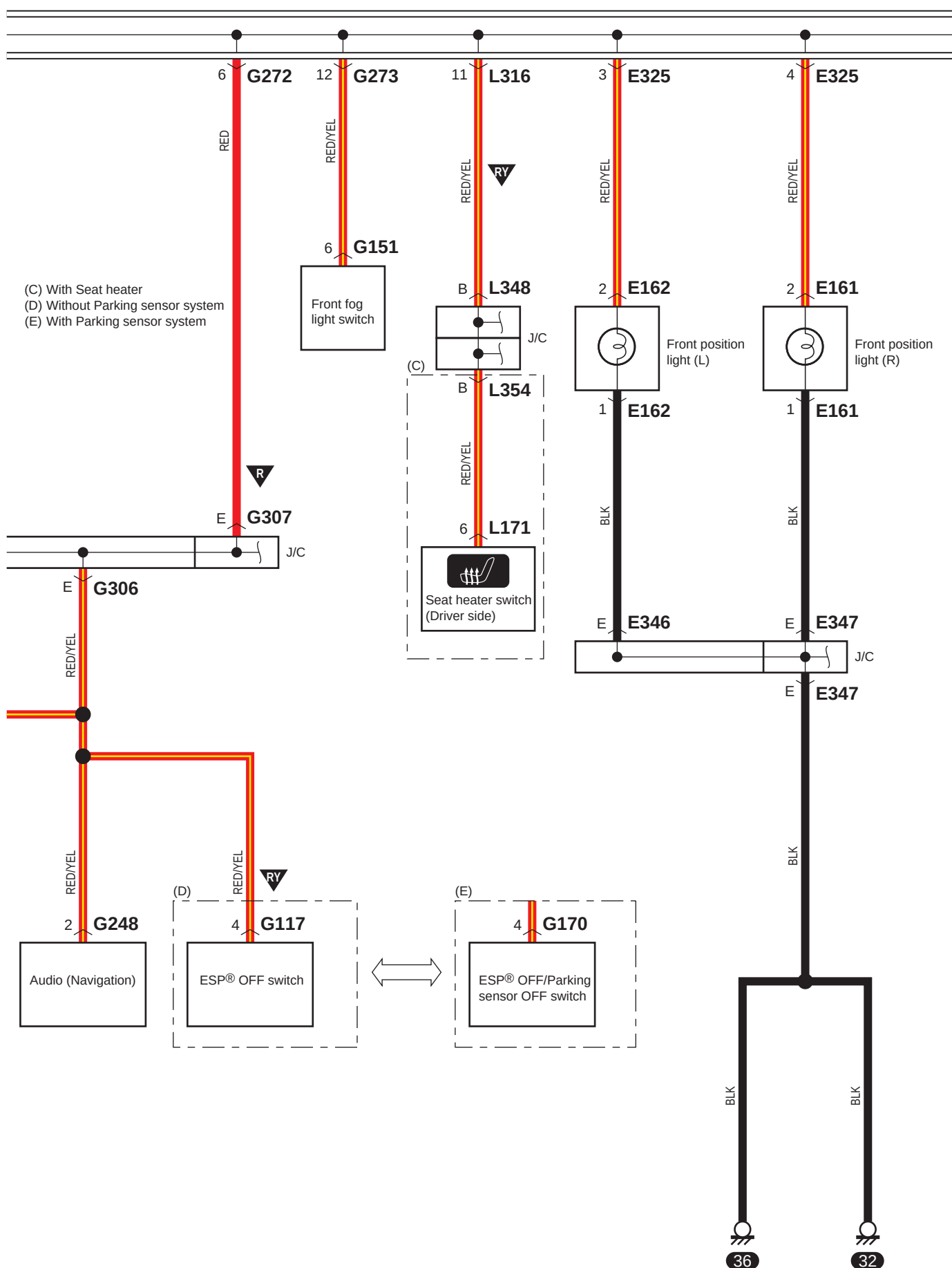
D-2-2 Helyzetjelző, hátsó, megvilágító és rendszámtábla lámpa kapcsolási rajza (nyomógombos motorindító rendszerrel)
