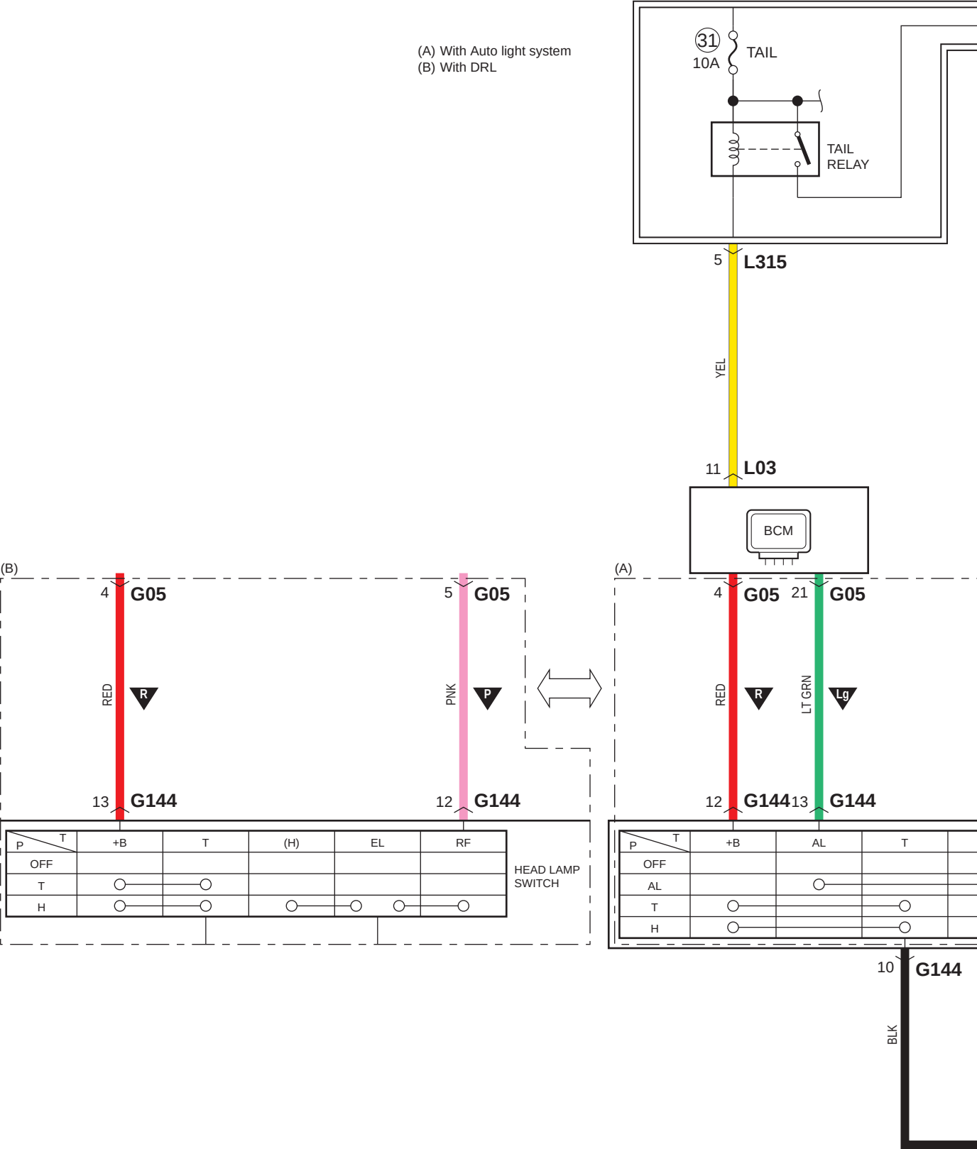
D-2-2 Helyzetjelző, hátsó, megvilágító és rendszámtábla lámpa kapcsolási rajza (nyomógombos motorindító rendszerrel)
