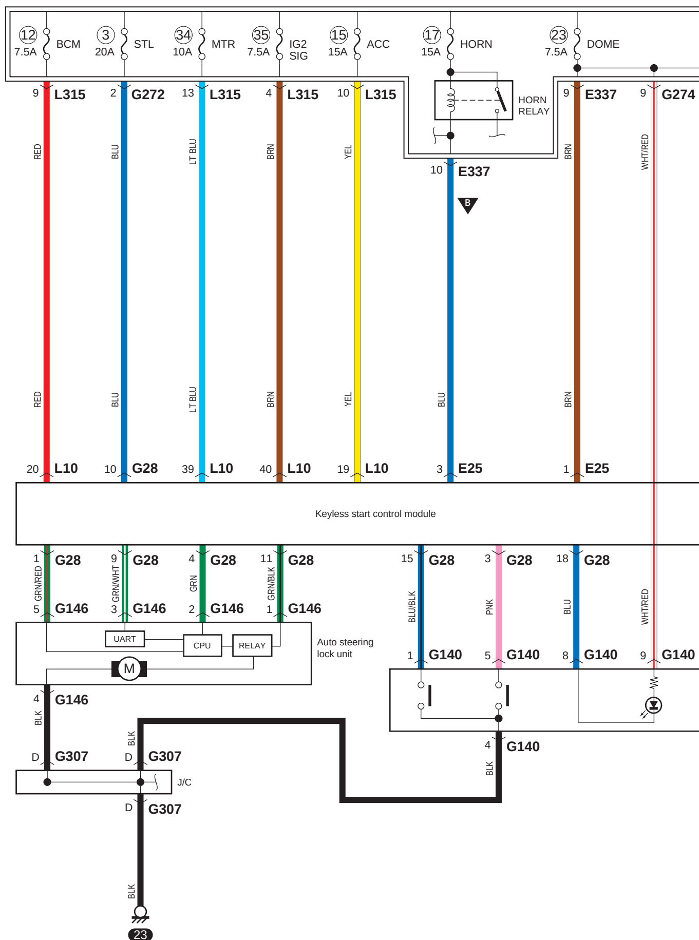
A-10 Schema elettrico del sistema di controllo sicurezza senza chiave (con sistema di avviamento motore a pulsante)
