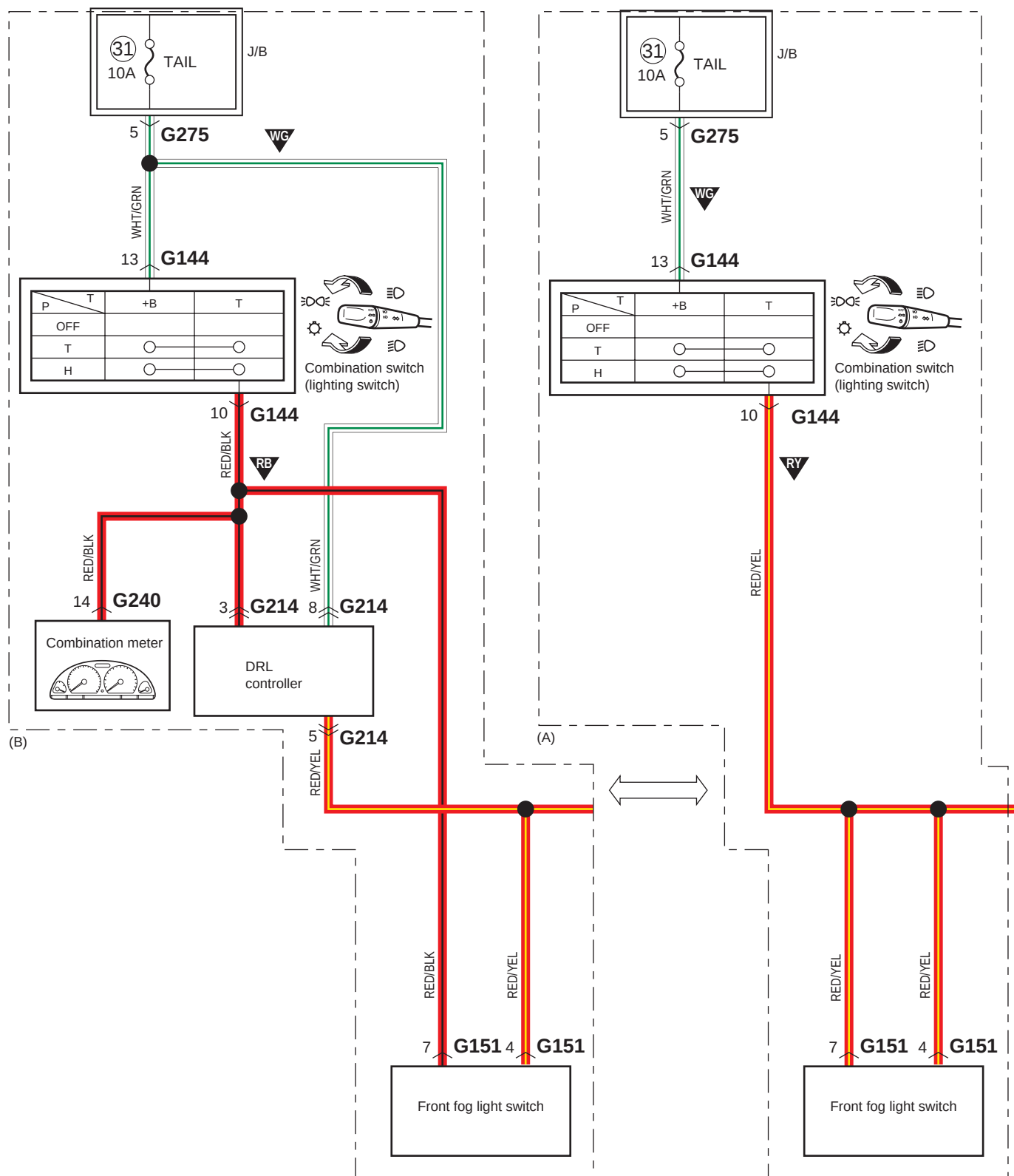
D-2-1 Schema elettrico del sistema luci di posizione anteriori, posteriori, illuminazione e luci targa (senza sistema di avviamento motore a pulsante)
