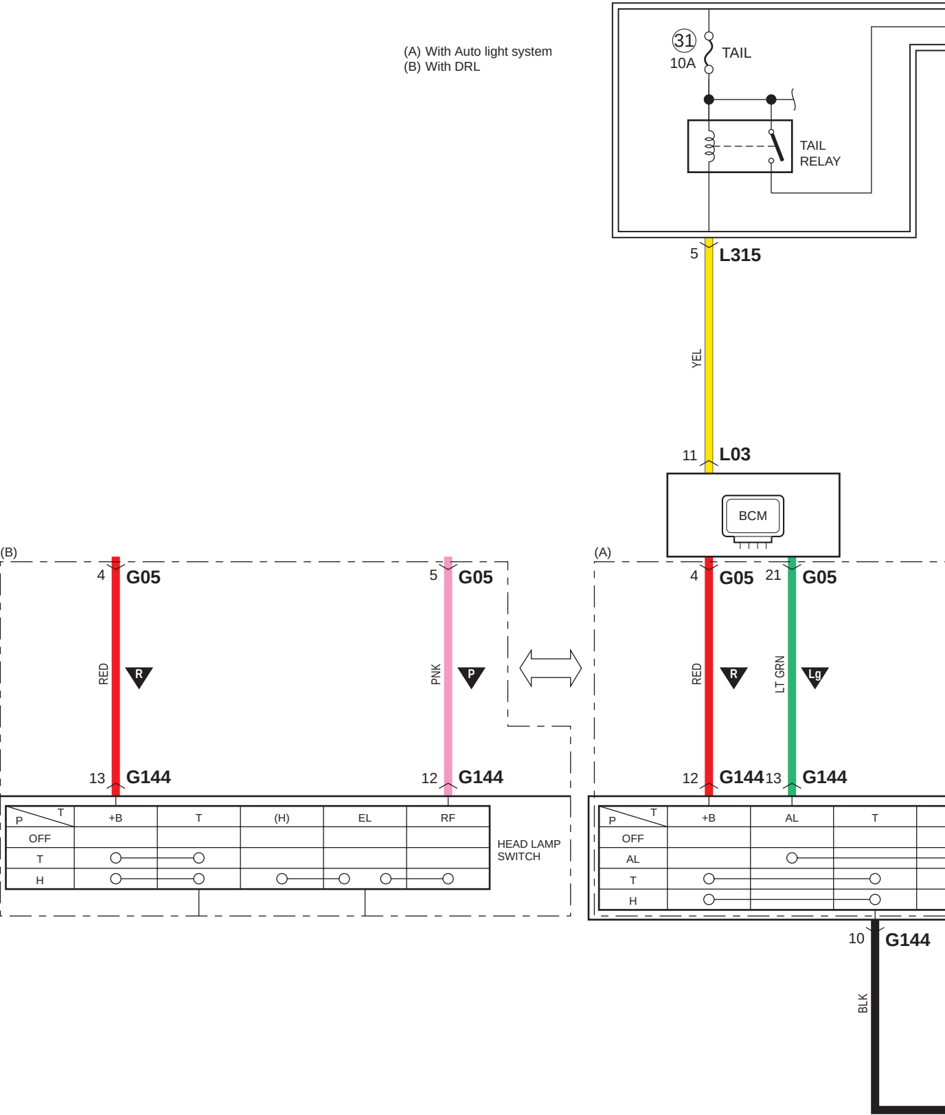
D-2-2 Schema elettrico del sistema luci di posizione anteriori, posteriori, illuminazione e luci targa (con sistema di avviamento motore a pulsante)
