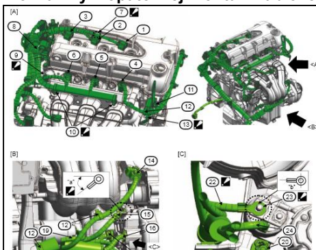
Poznámky k opätovnej montáži káblového zväzku
