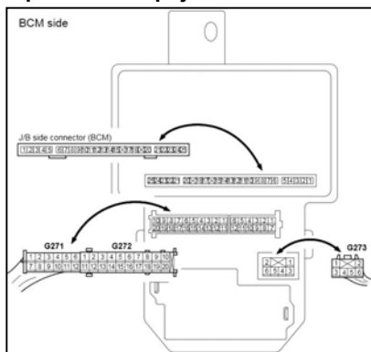
Usporiadanie spojovacieho bloku
