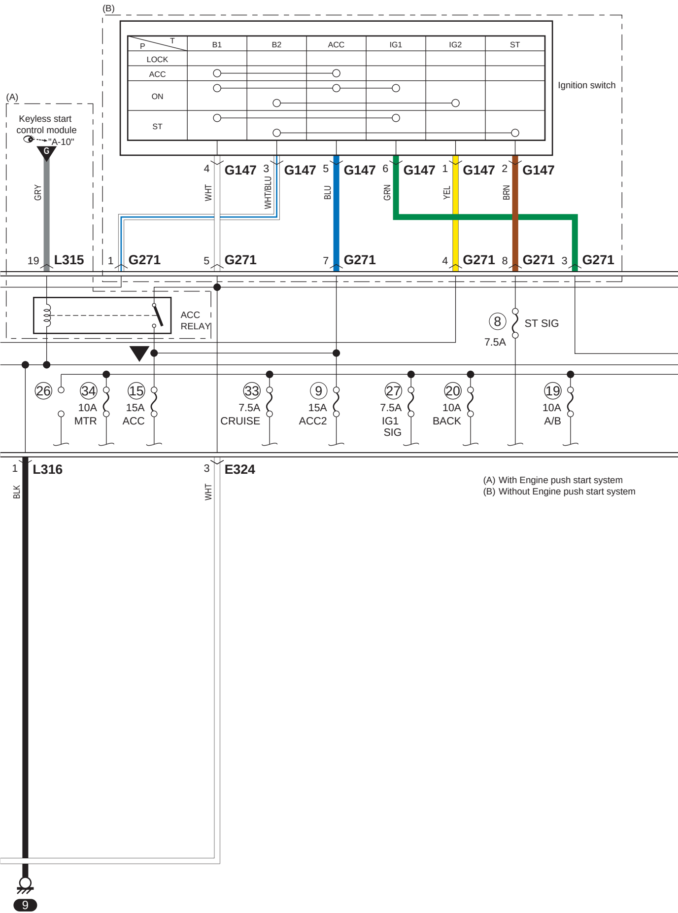
P-1-1 Schéma napájania (model s benzínovým motorom)
