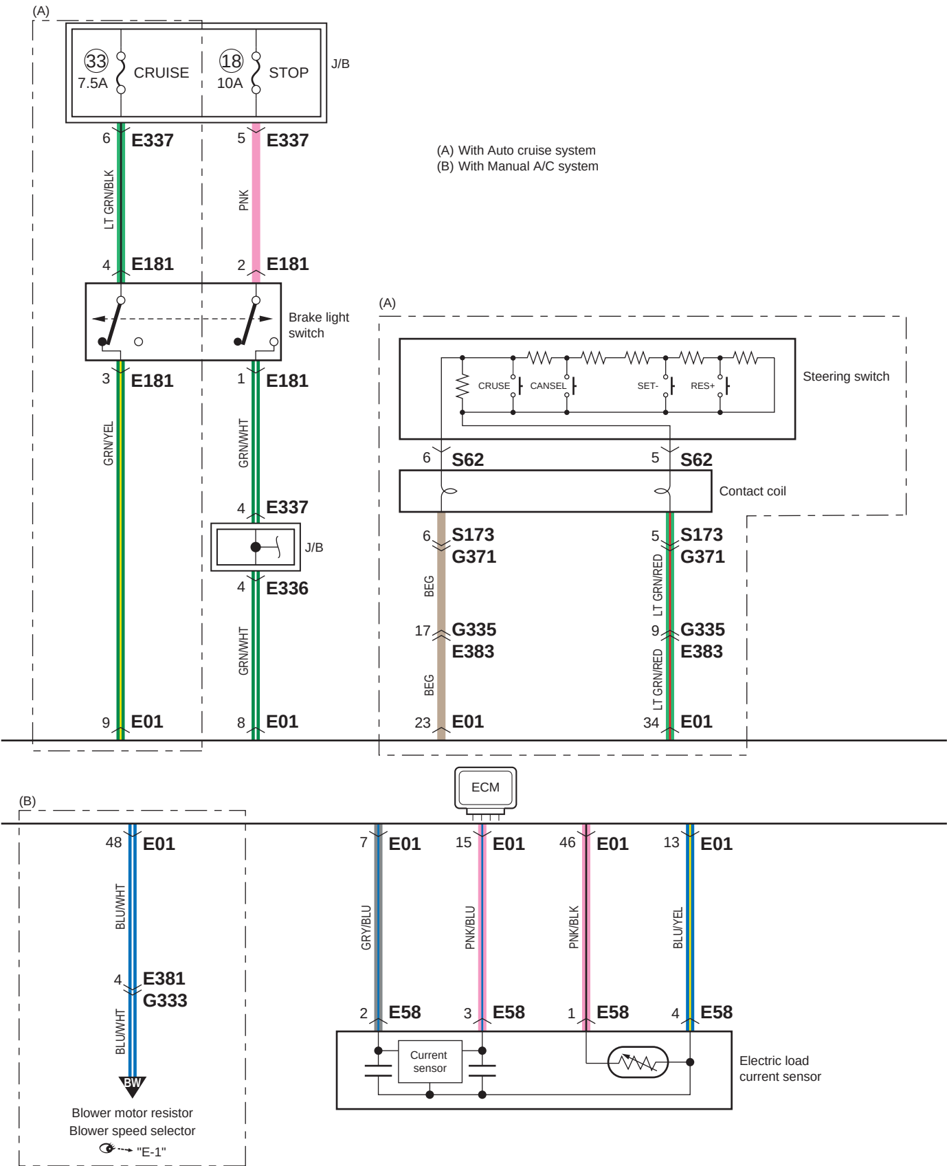
A-5-1 Schéma zapojenia obvodu riadiaceho systému motora a klimatizácie (model s benzínovým motorom)
