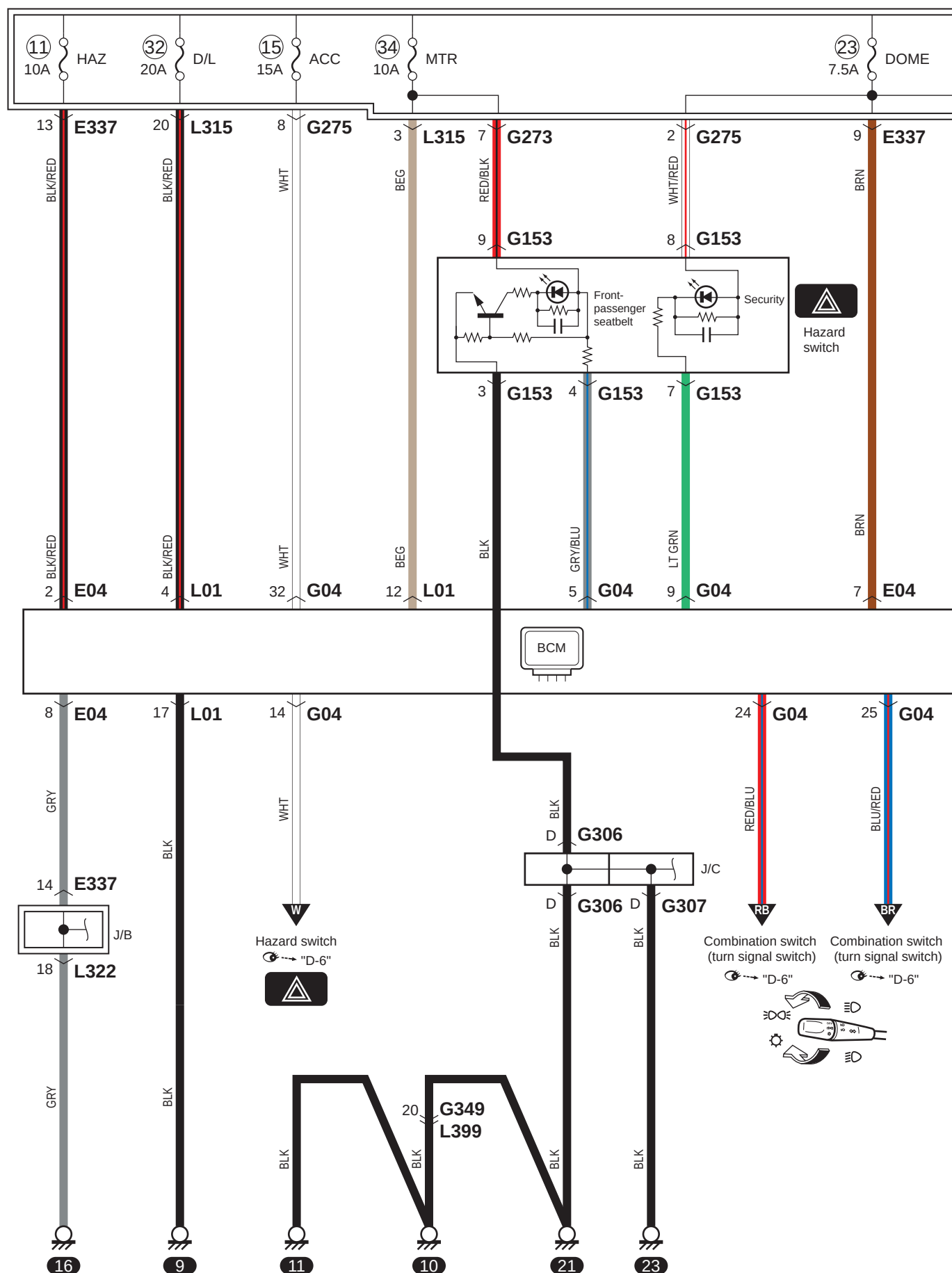
A-8-1 Schéma zapojenia obvodu riadiaceho systému karosérie (bez stláčacieho štartovacieho systému motora)
