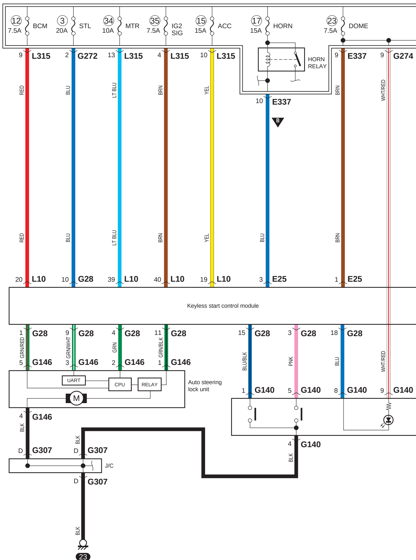
A-10 Schéma zapojenia obvodu bezklúčového bezpečnostného riadiaceho systému (so stláčacím štartovacím systémom motora)
