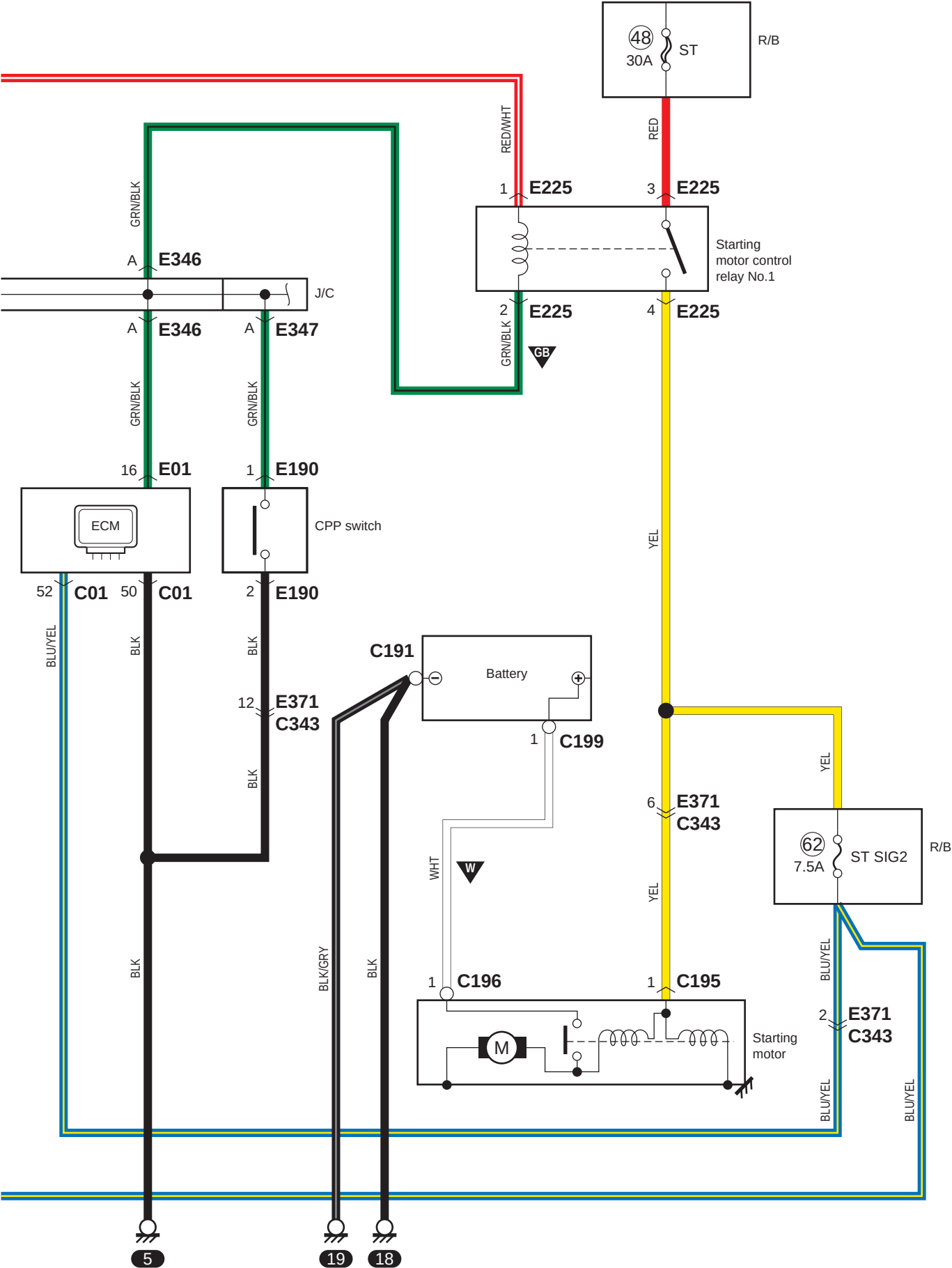
A-1-2 Diagrama del circuito del sistema de arranque (modelos de gasolina con sistema de arranque por pulsación del motor)
