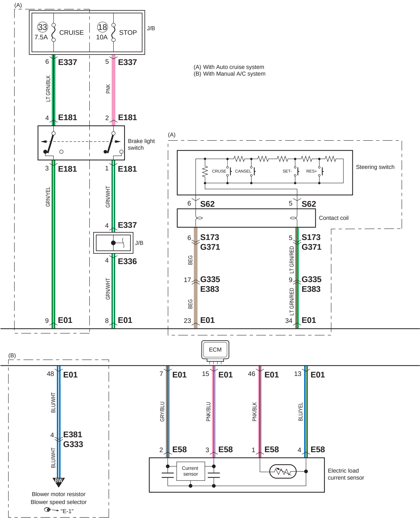
A-5-1 Diagrama del circuito del sistema de control del A/C y del motor (modelos de gasolina)
