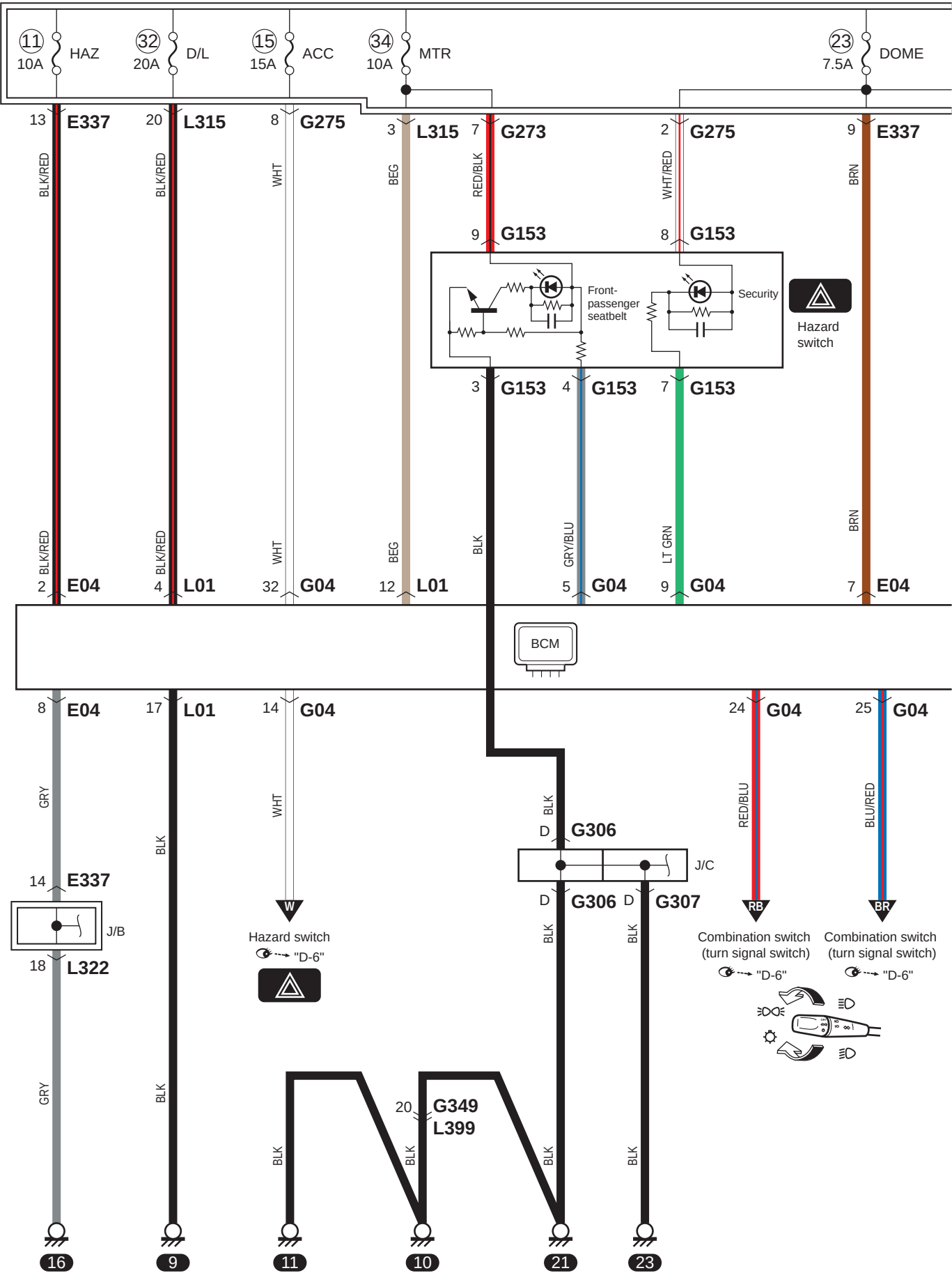
A-8-1 Diagrama del circuito del sistema de control de la carrocería (sin sistema de arranque por pulsación del motor)
